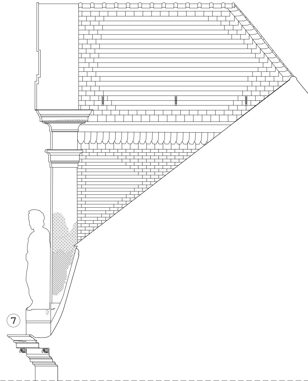
RECHTERZIJAANZICHT MIDDENRISALIET bestaande toestand - schaal 1 : 100
