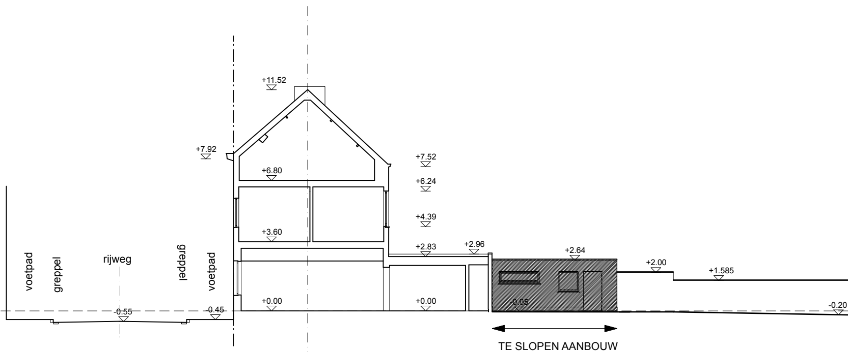
TERREINPROFIEL bestaand
