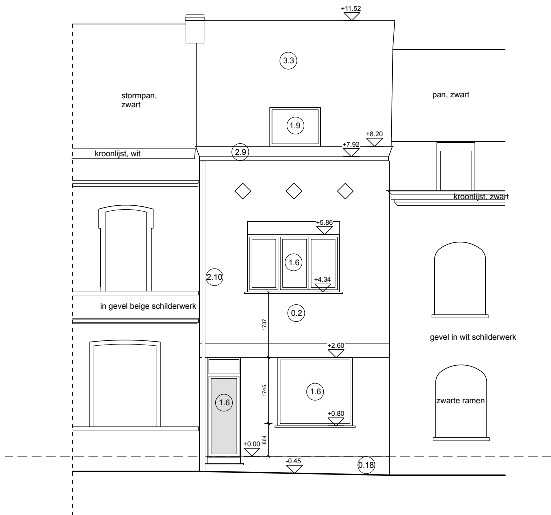
VOORGEVEL nieuw
