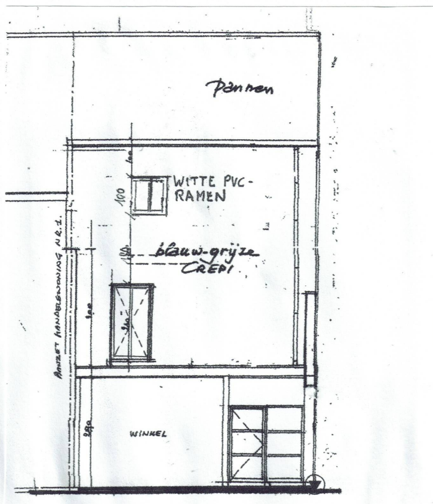
ACHTERGEVEL BESTAANDE TOESTAND 1/100 (wijzig niet)
