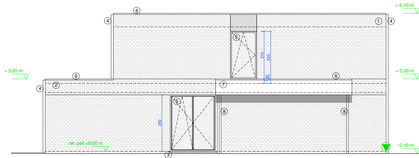
ZIJGEVEL LINKS
