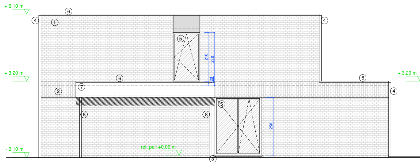
ZIJGEVEL RECHTS
