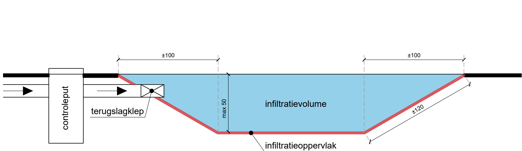
principesnede infiltratievoorziening (WADI) - (schaal 1/20)
