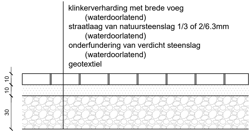
schematische opbouw waterdoorlatende verharding - (schaal 1/20)
