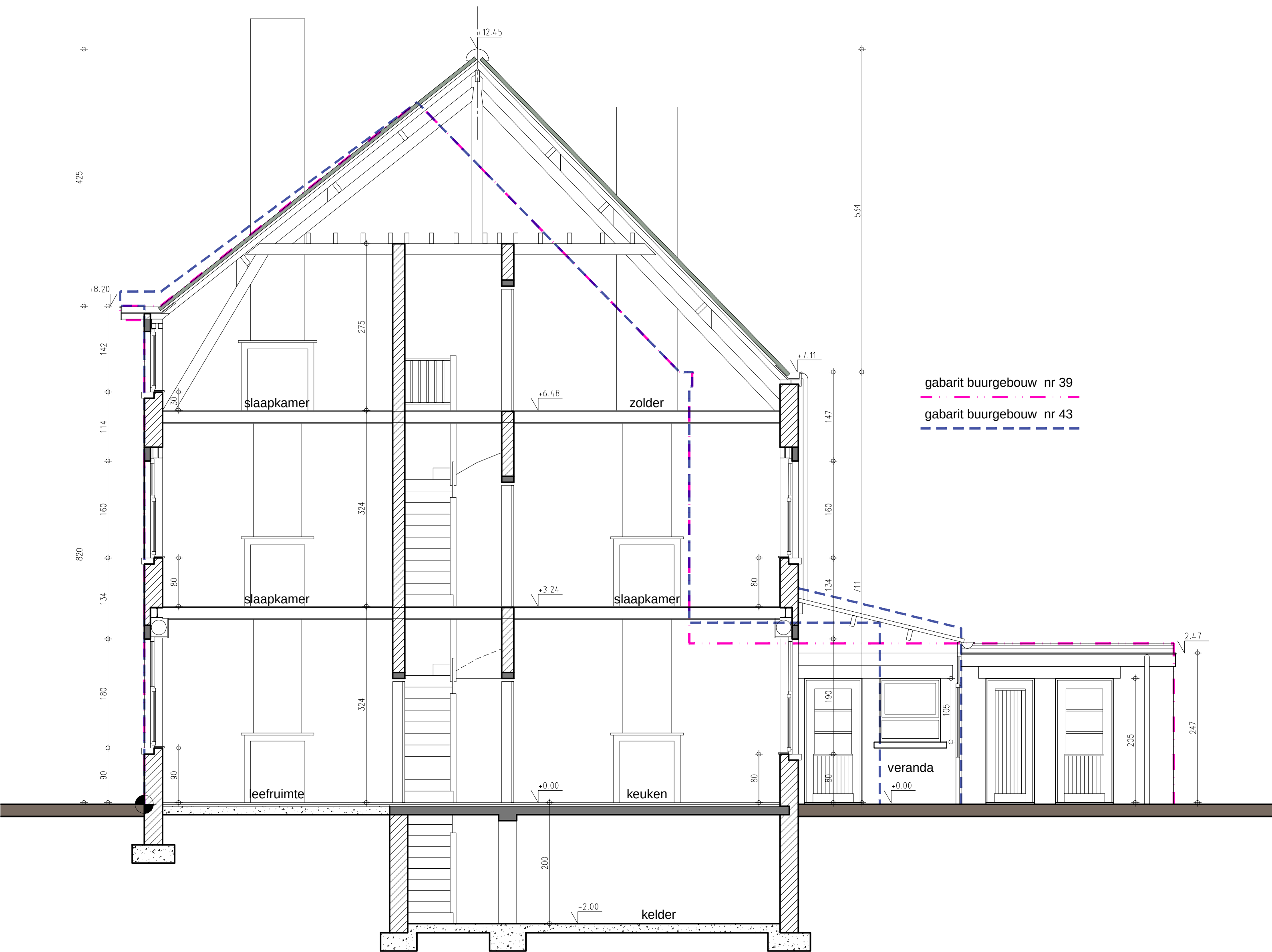
DOORSNEDE 1-1 - bestand 1/50
