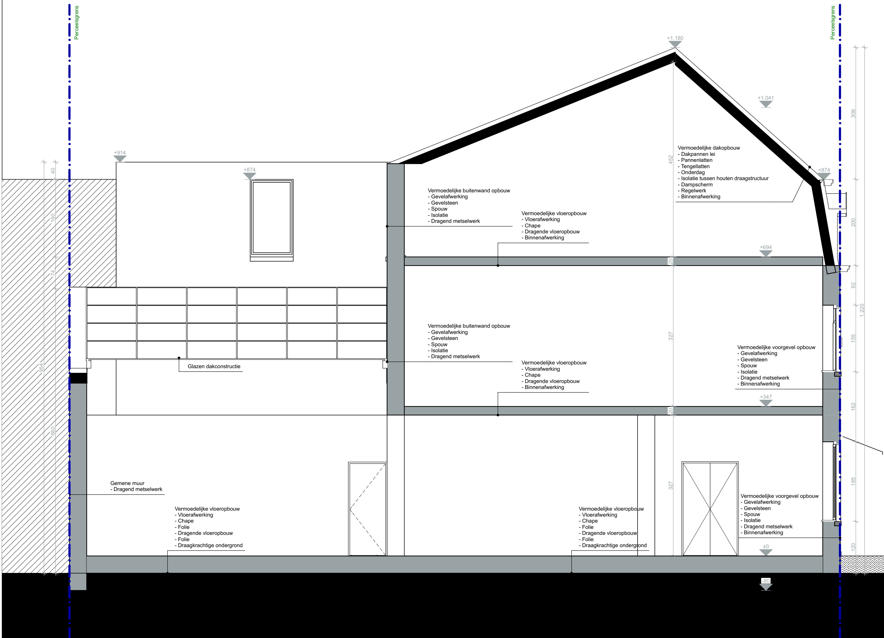
DOORSNEDE BB NIEUWE TOESTAND
