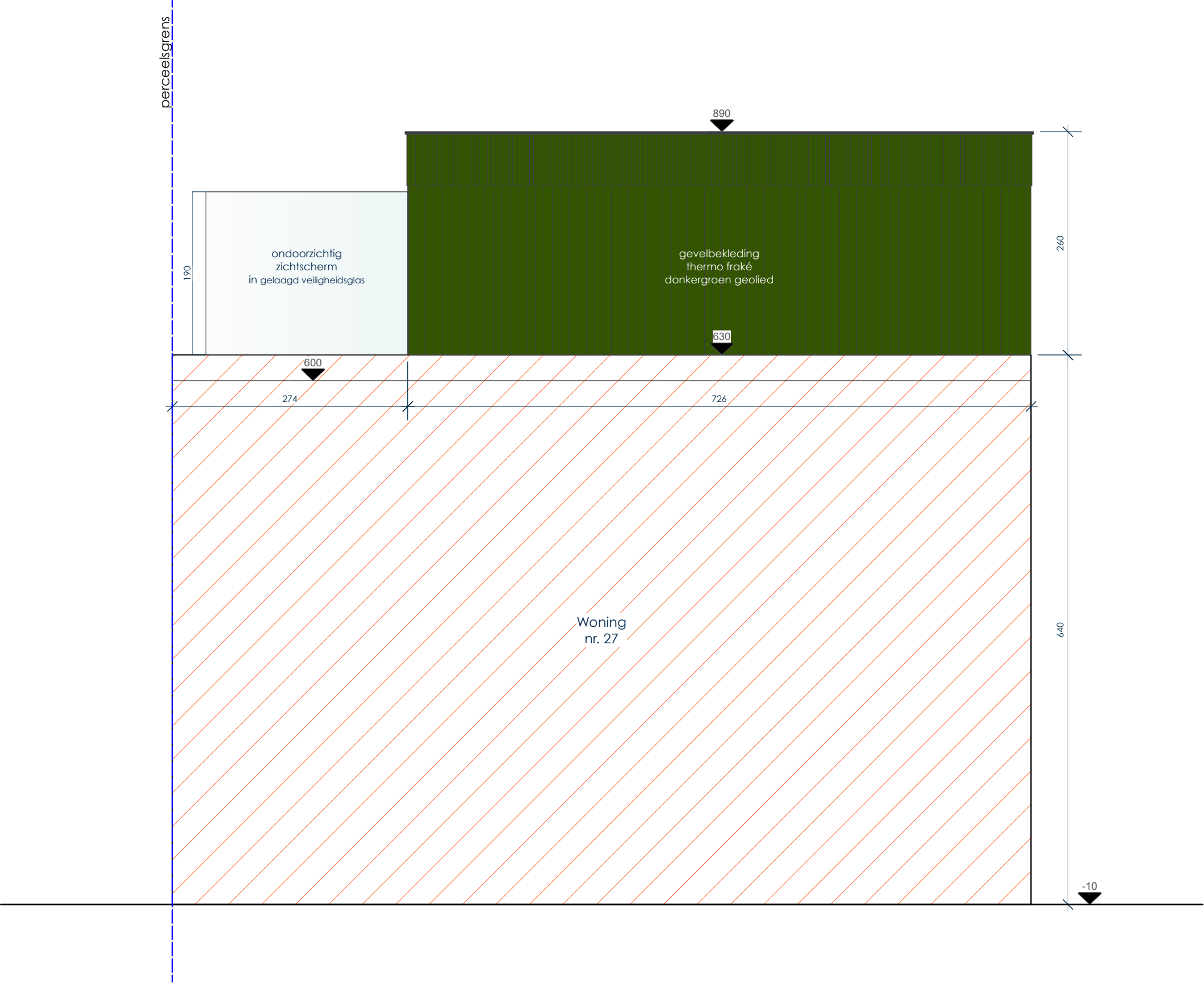
ZIJGEVEL RECHTS - nieuwe toestand - schaal 1/50
