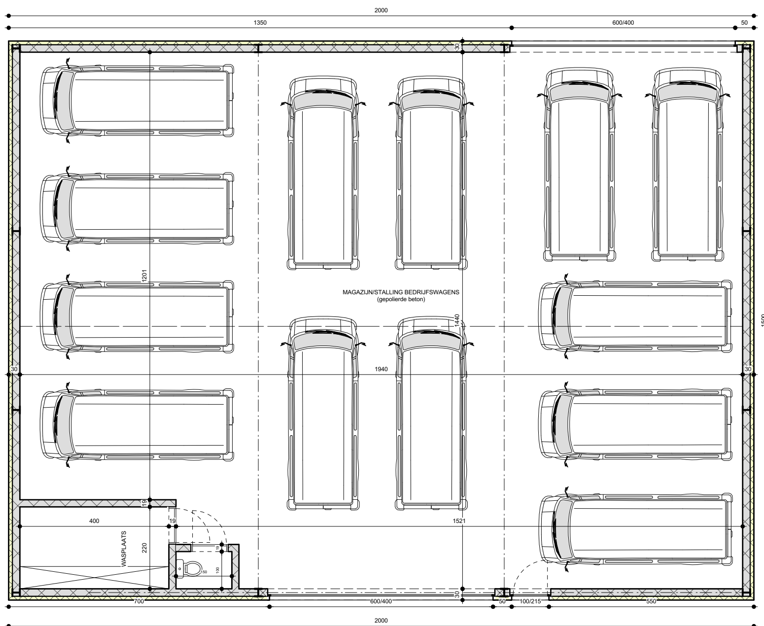
GRONDPLAN 300m²
