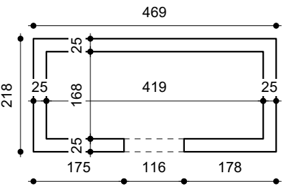
GRONDPLAN hondenhok
