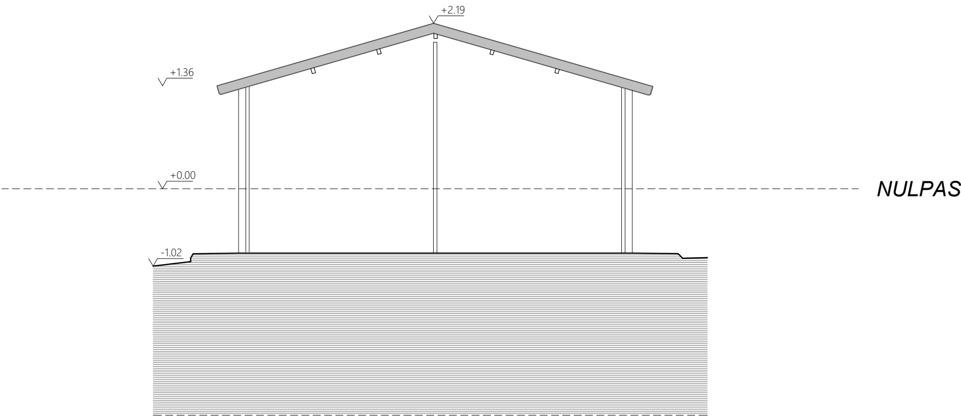
BG3: ACHTERGEVEL
