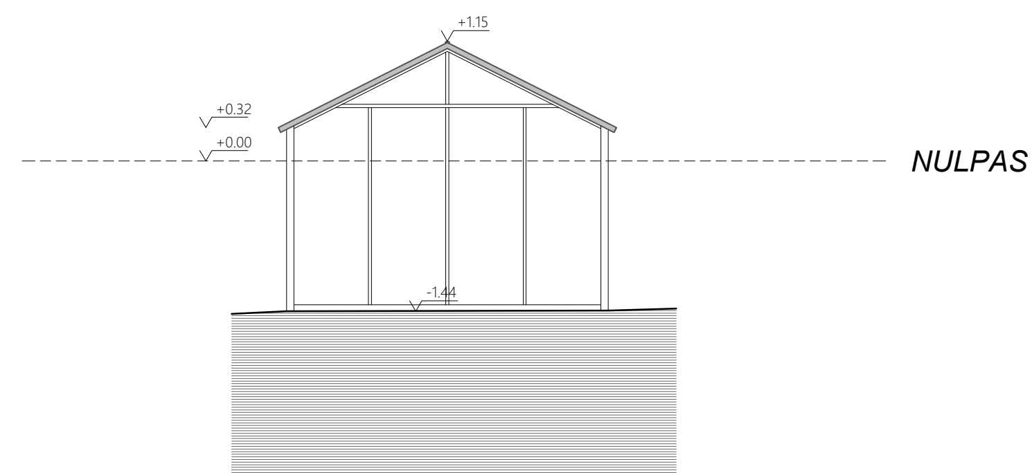
BG1: ACHTERGEVEL
