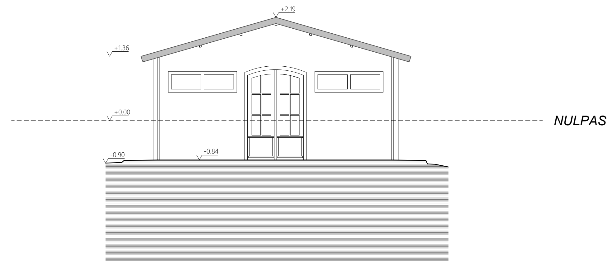
BG3: VOORGEVEL
