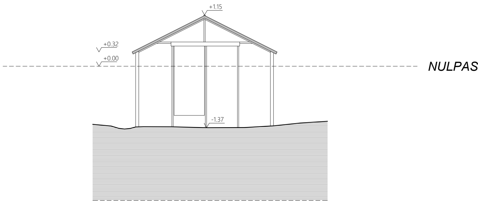
BG1: VOORGEVEL
