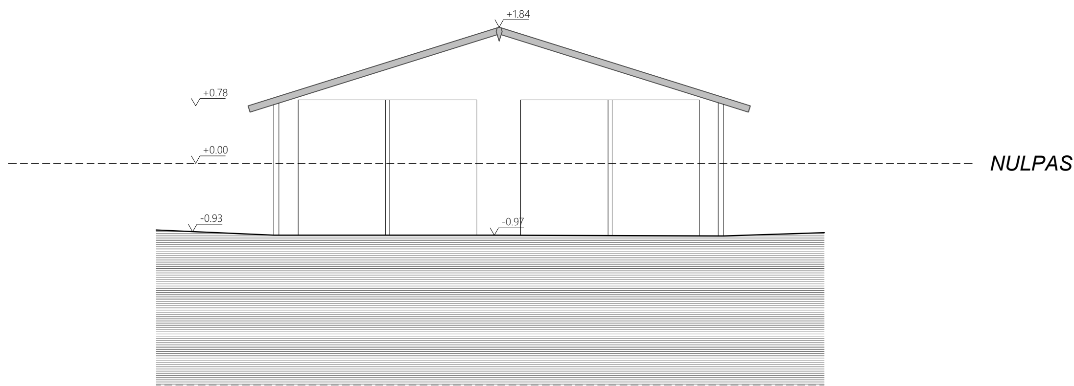
BG2: VOORGEVEL
