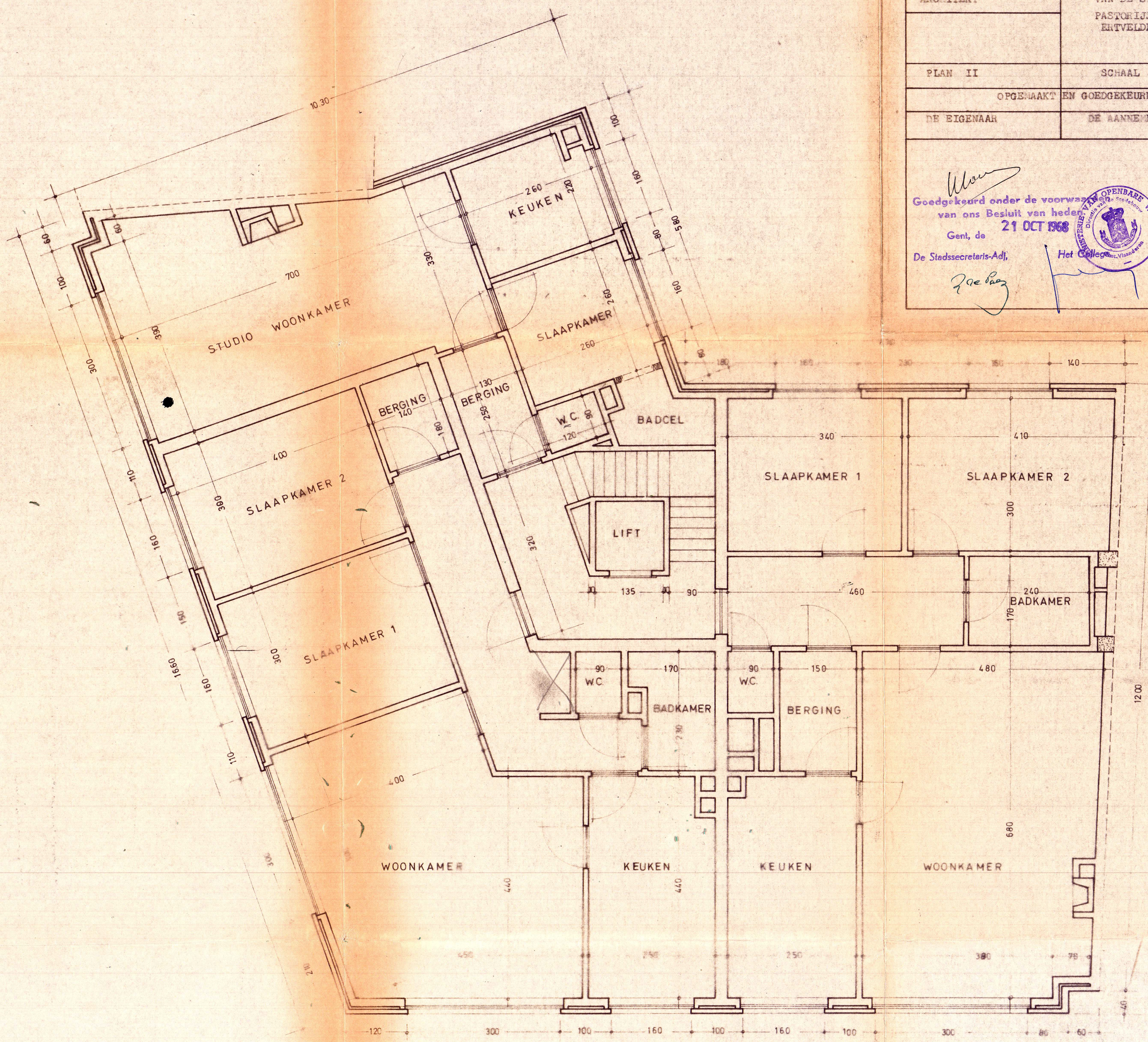
PLAN TWEEDE EN DERDE VERDIEPING
