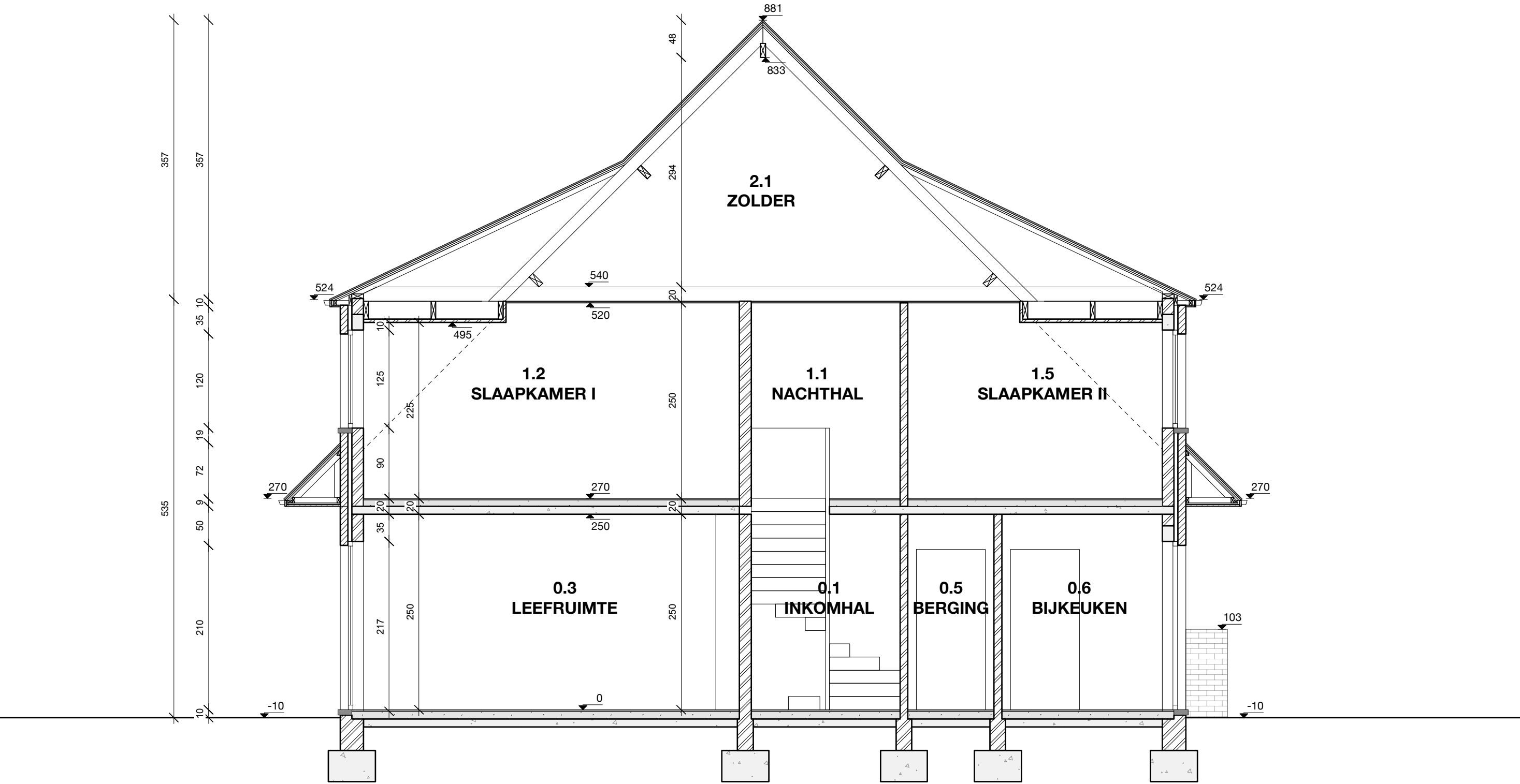
SNEDE AA bestaande toestand schaal 1/50
