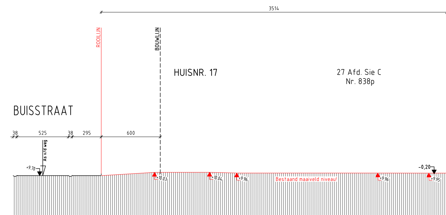
TERREINPROFIEL 1/200 BESTAANDE TOESTAND
