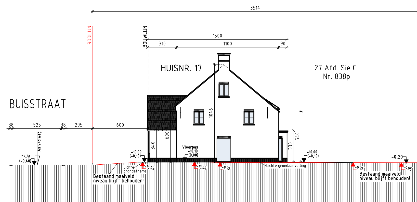
TERREINPROFIEL 1/200 NIEUWE TOESTAND
