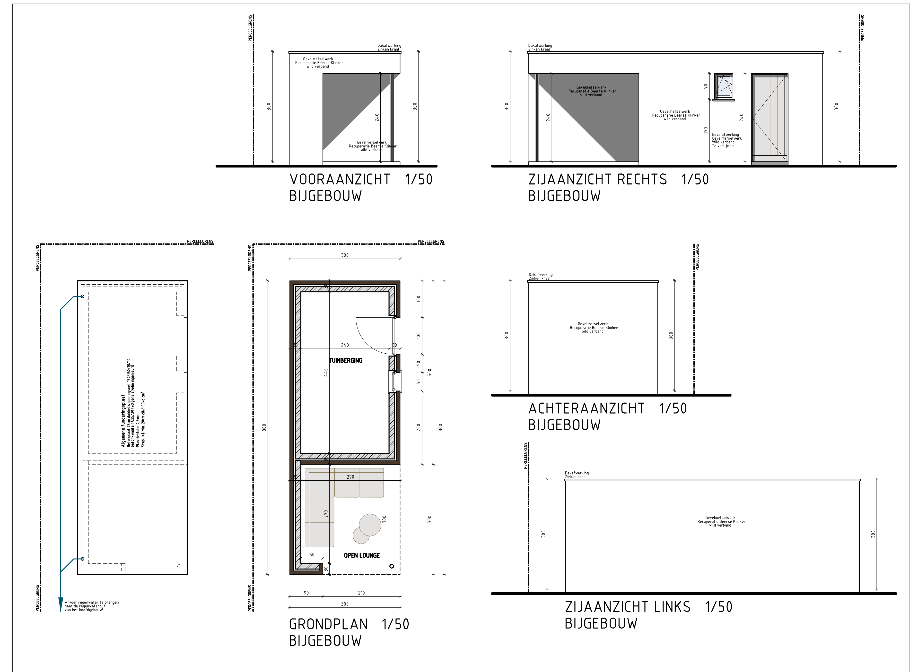
PLAN BIJGEBOUW SCHAAL 1/50
