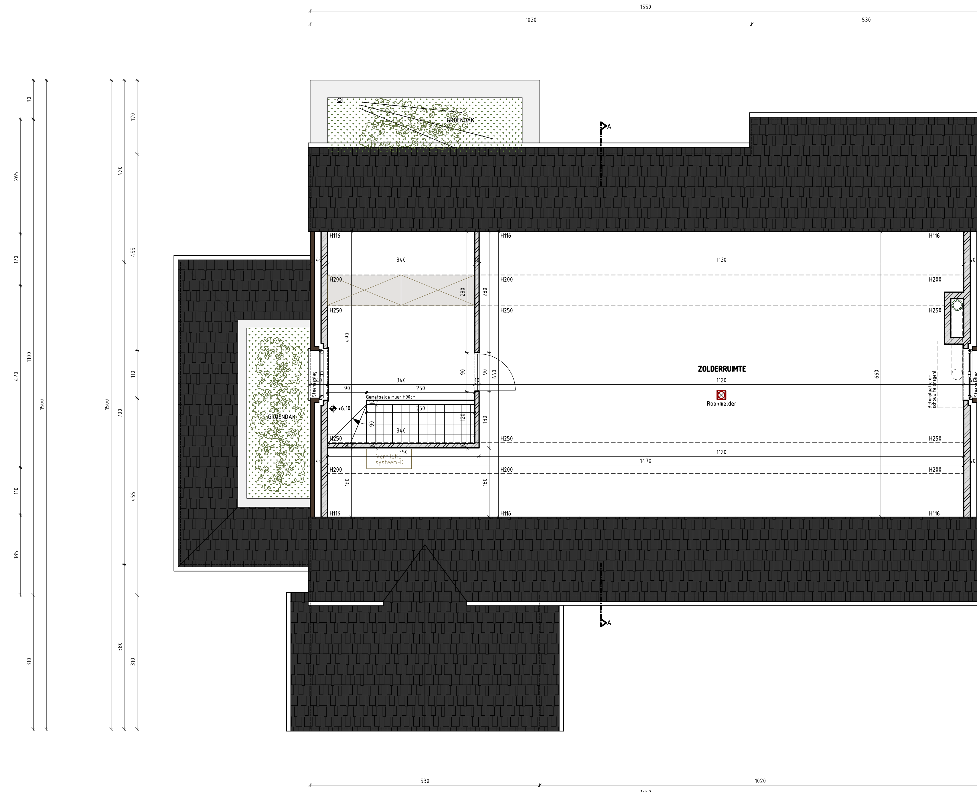
PLAN ZOLDERVERDIEPING SCHAAL 1/50
