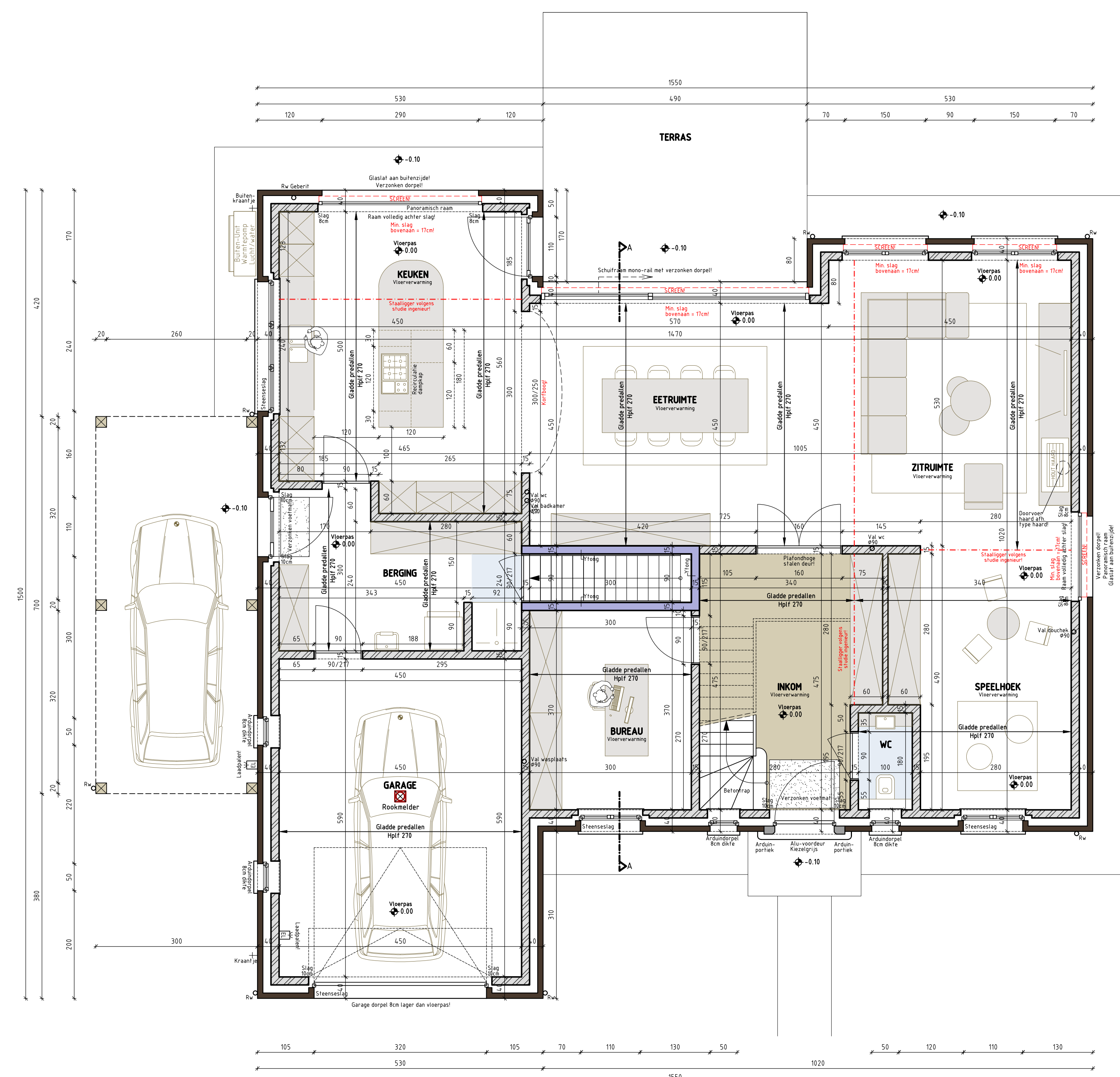
PLAN GELIJKVLOERS SCHAAL 1/50
