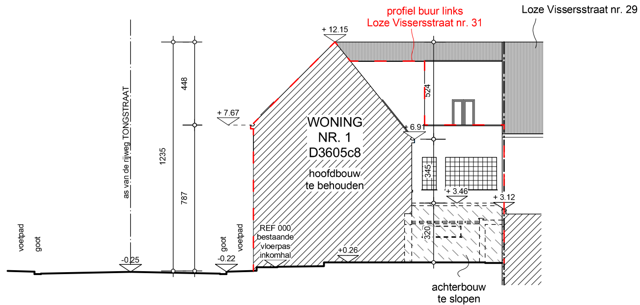
TERREINPROFIEL AB BESTAANDE TOESTAND schaal 1/200
