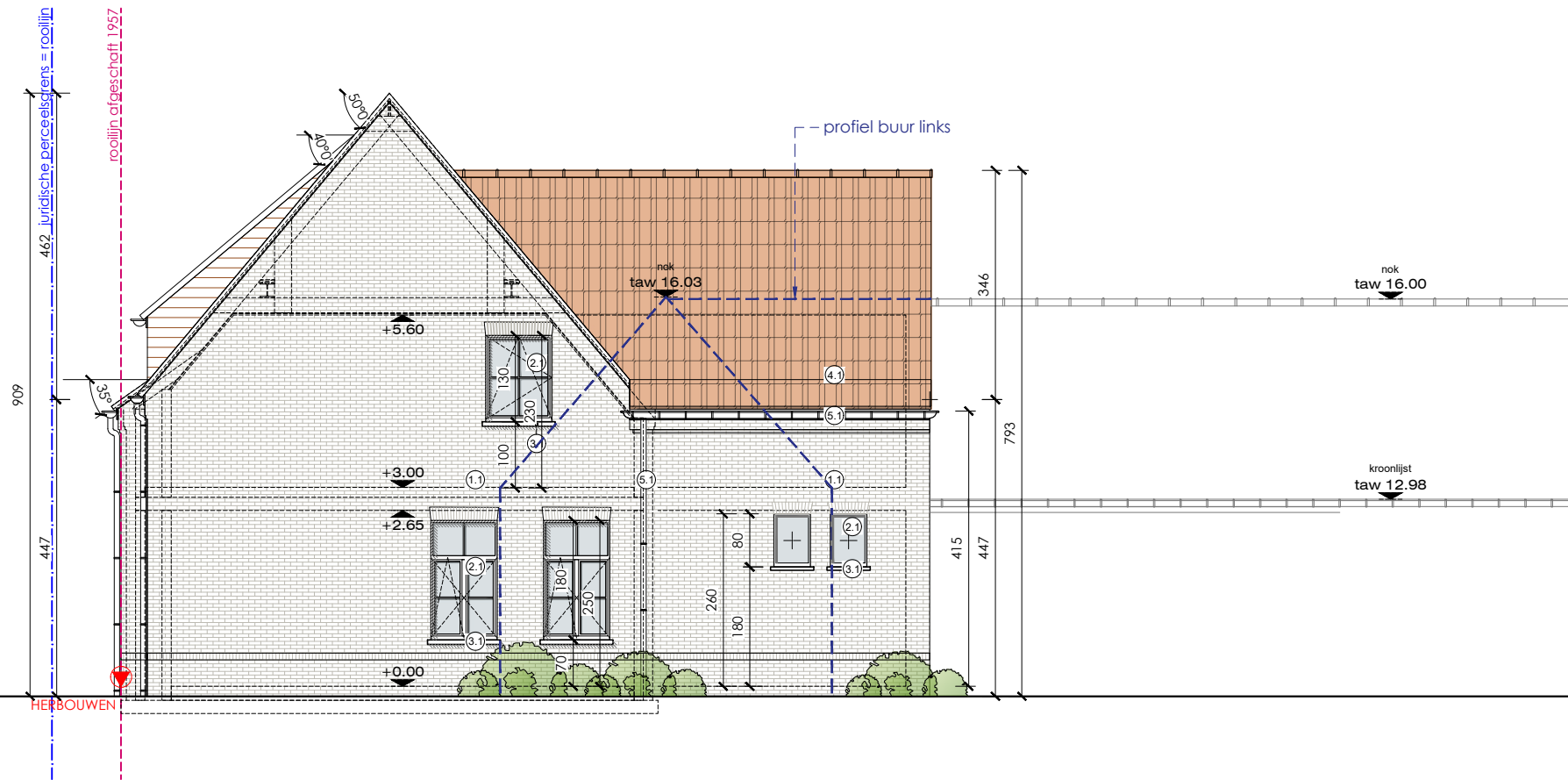
ZIJGEVEL RECHTS
