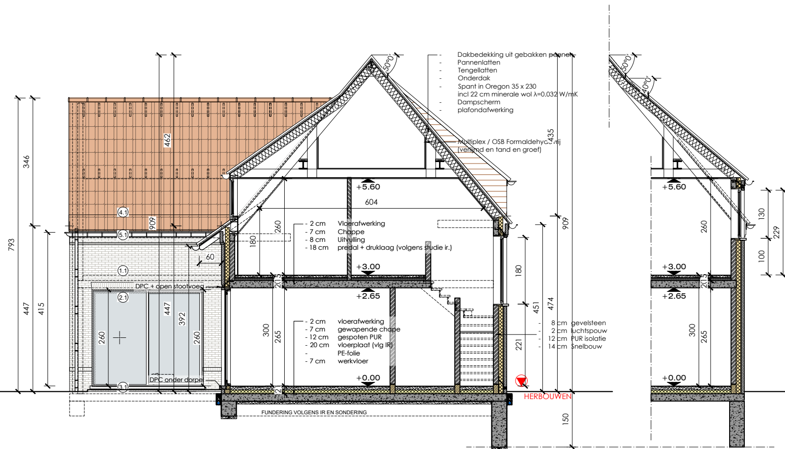
DOORSNEDE AA
