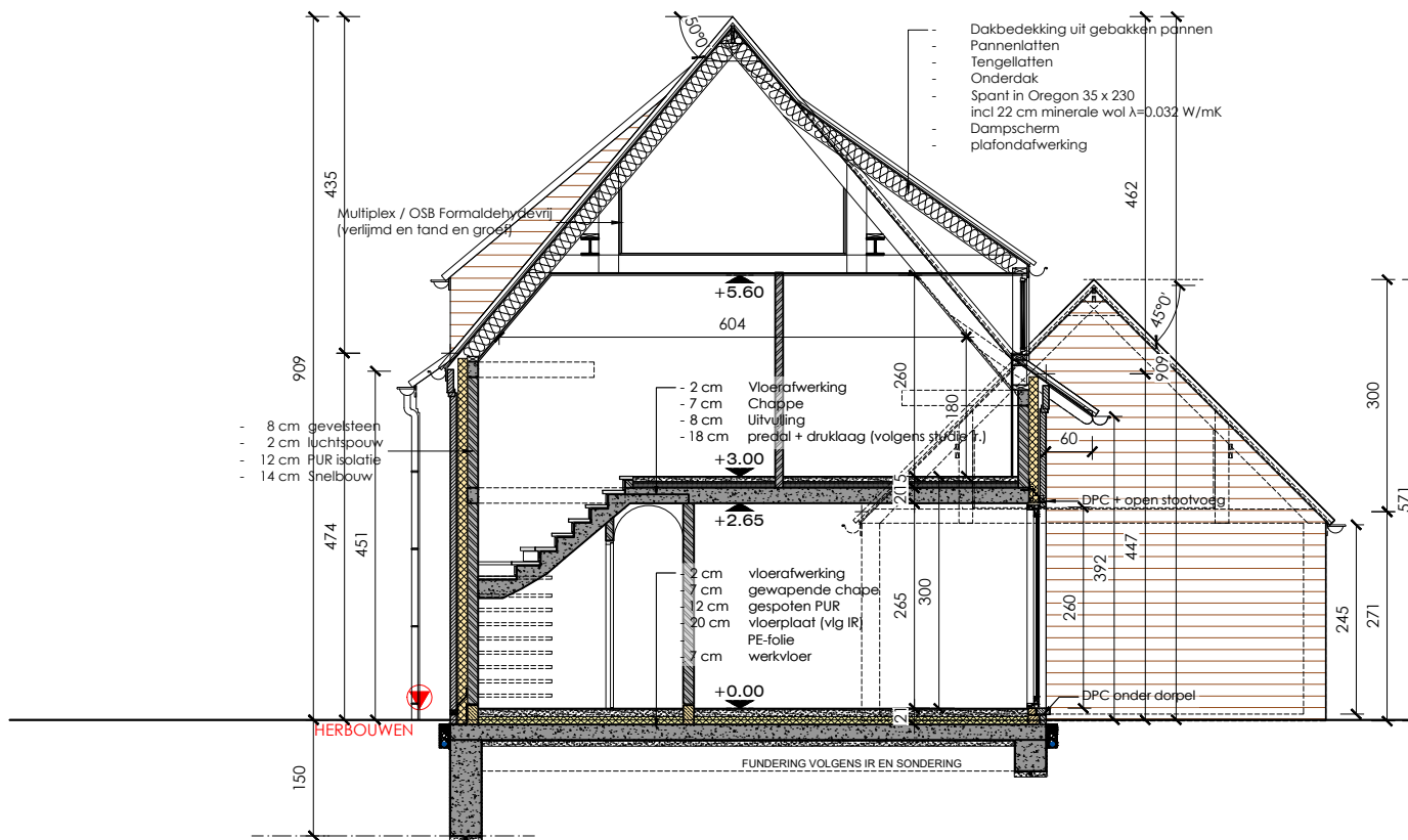
DOORSNEDE BB
