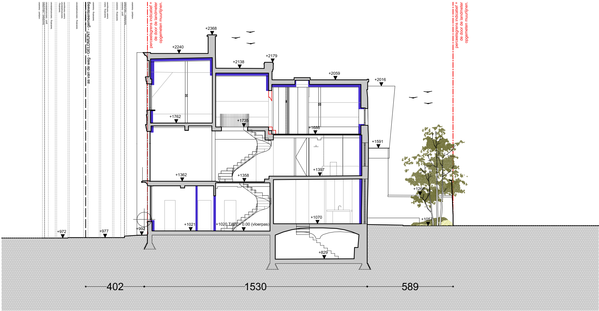
TERREINPROFIEL AA' - nieuwe toestand 0 2 10
