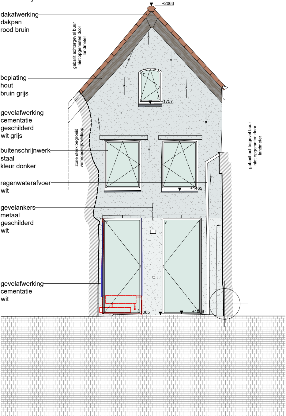
ACHTERGEVEL - OOST - nieuwe toestand
