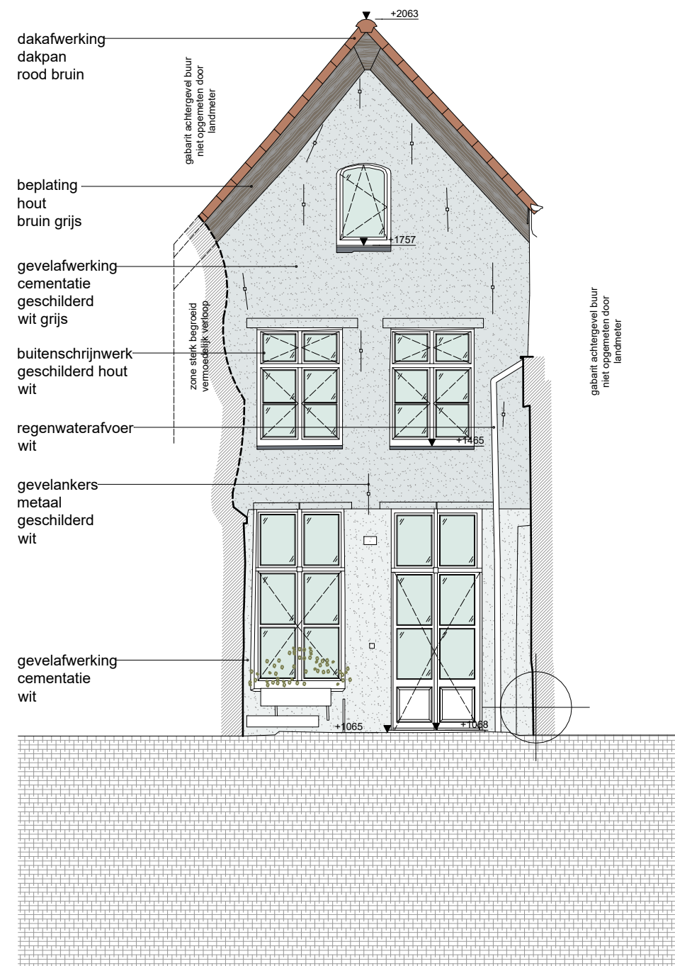
ACHTERGEVEL - OOST - bestaande toestand
