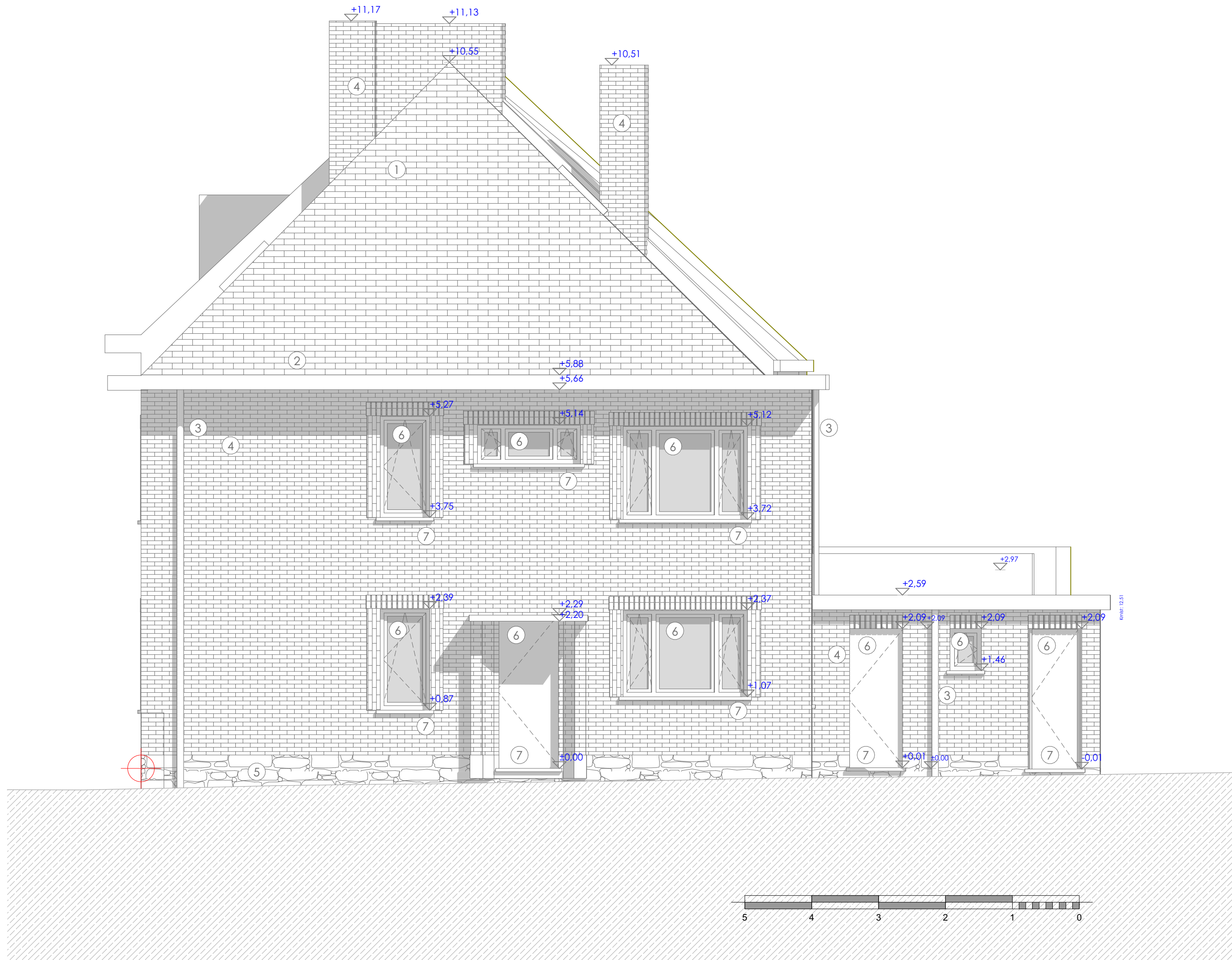
gevel rechts bestaand
