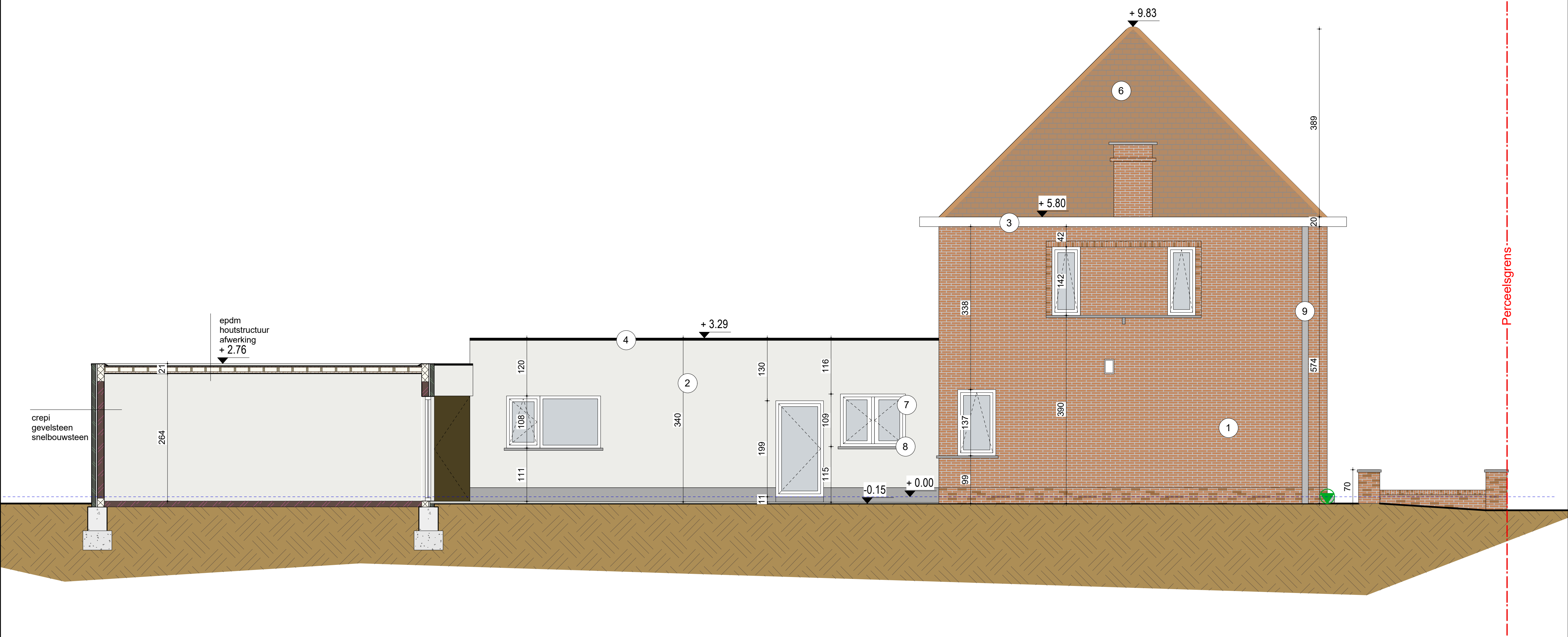
Zijgevel links BT Schaal: 1:50
