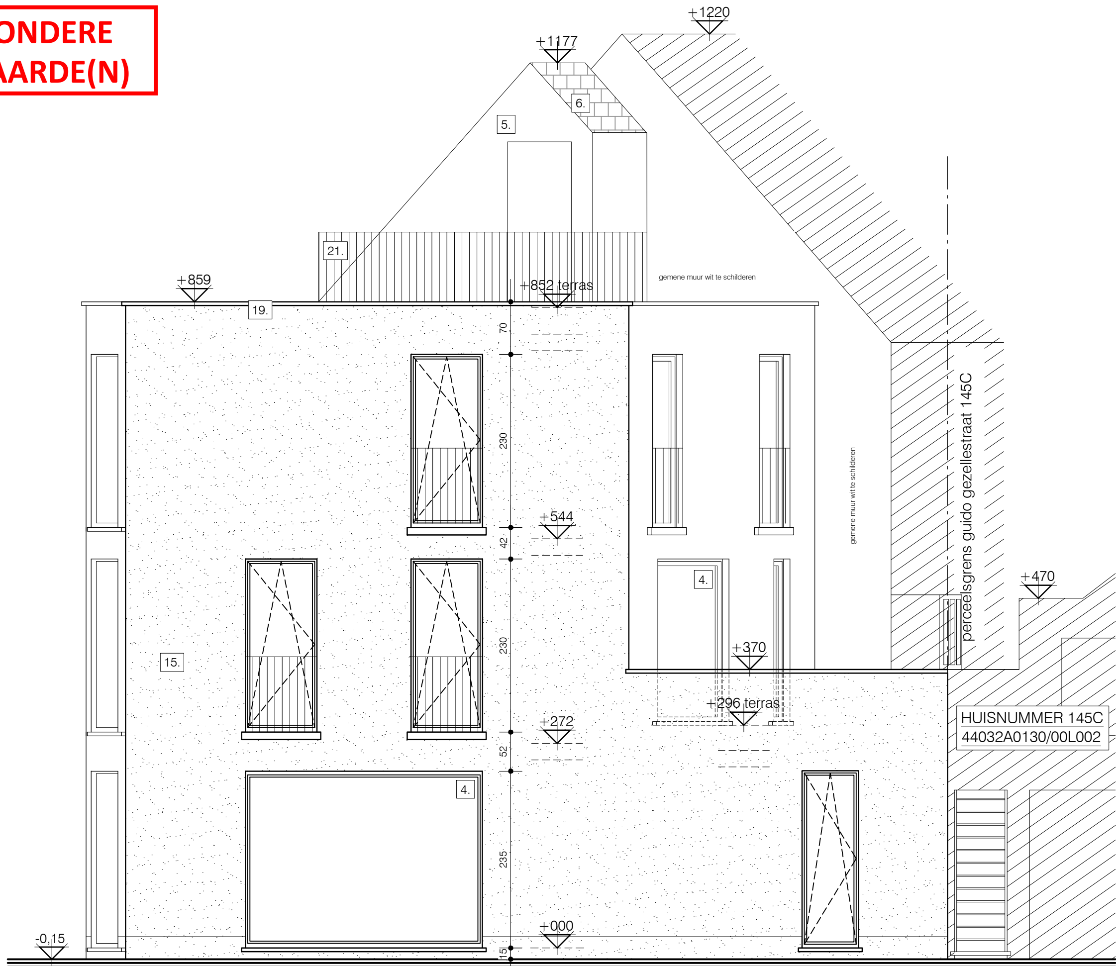
NIEUWE TOESTAND_RECHTERZIJGEVEL schaal: 1/50 - maatvoering in cm
