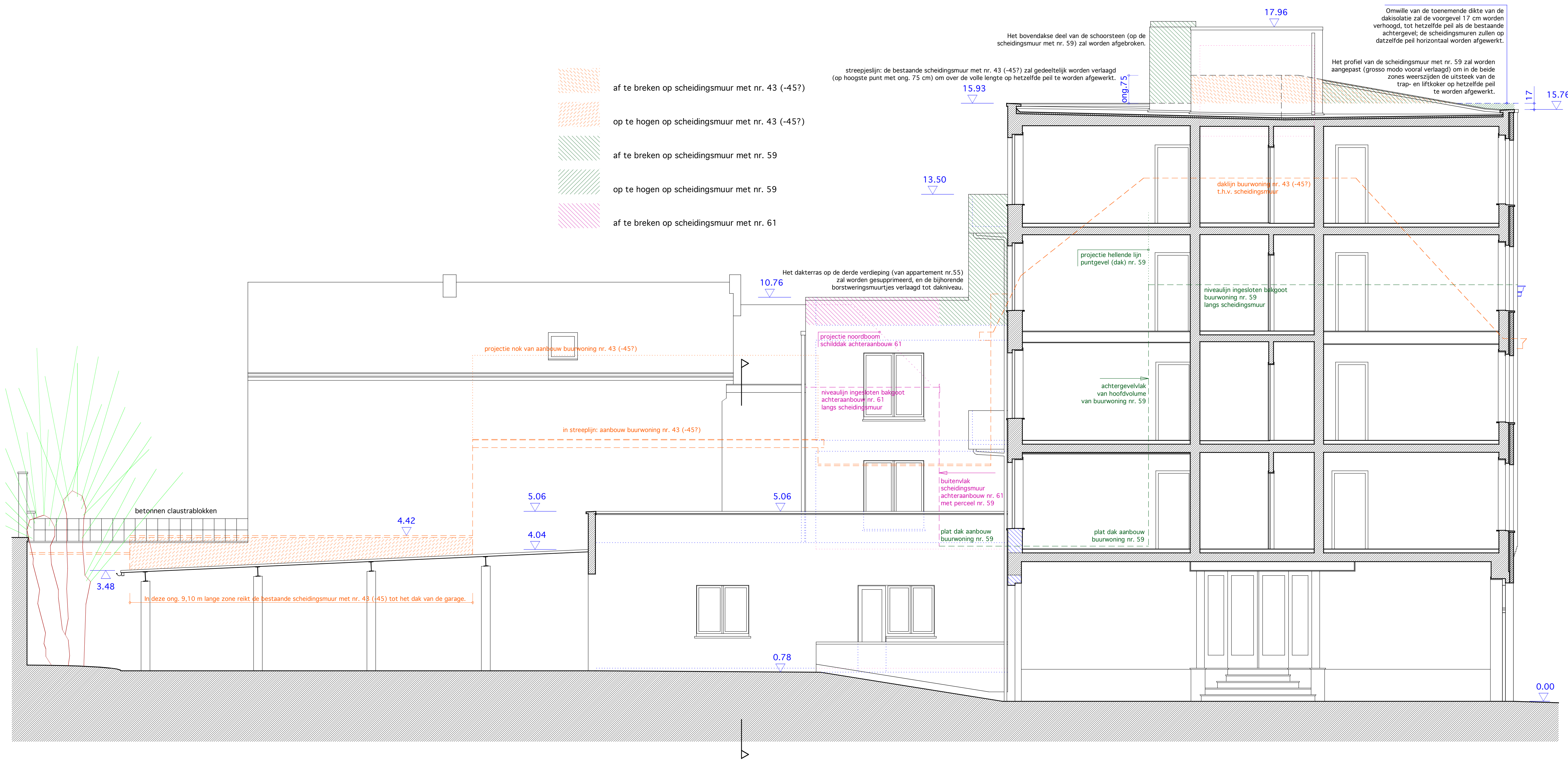
SLEEPSTRAAT (47-) 49-57, 9000 GENT * 1/50 TERREINPROFIEL t.h.v. DOORRIT, BESTAANDE TOESTAND
