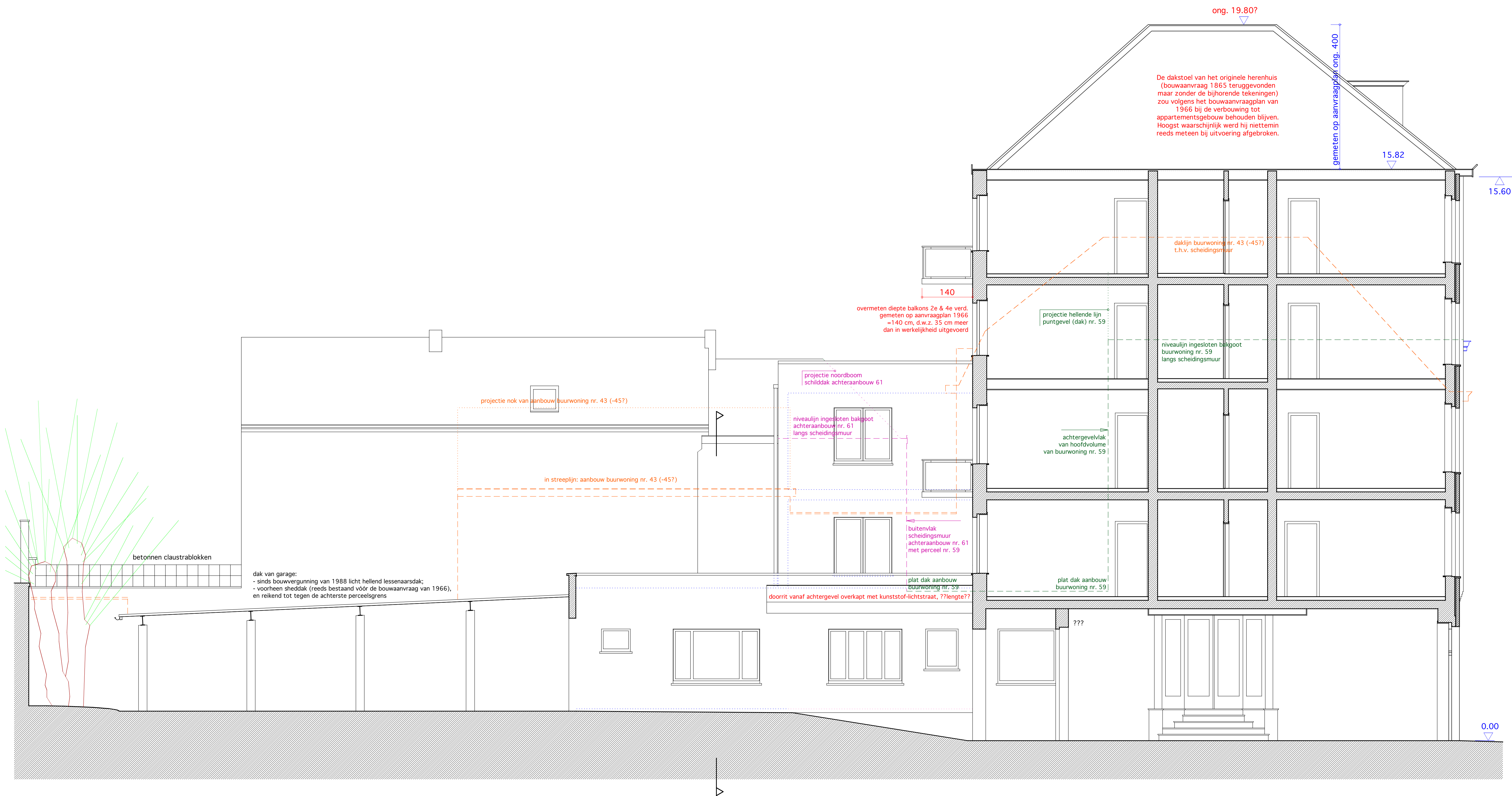
SLEEPSTRAAT (47-) 49-57, 9000 GENT * 1/50 TERREINPROFIEL t.h.v. DOORRIT, SIMULATIE van VERGUNDE TOESTAND
