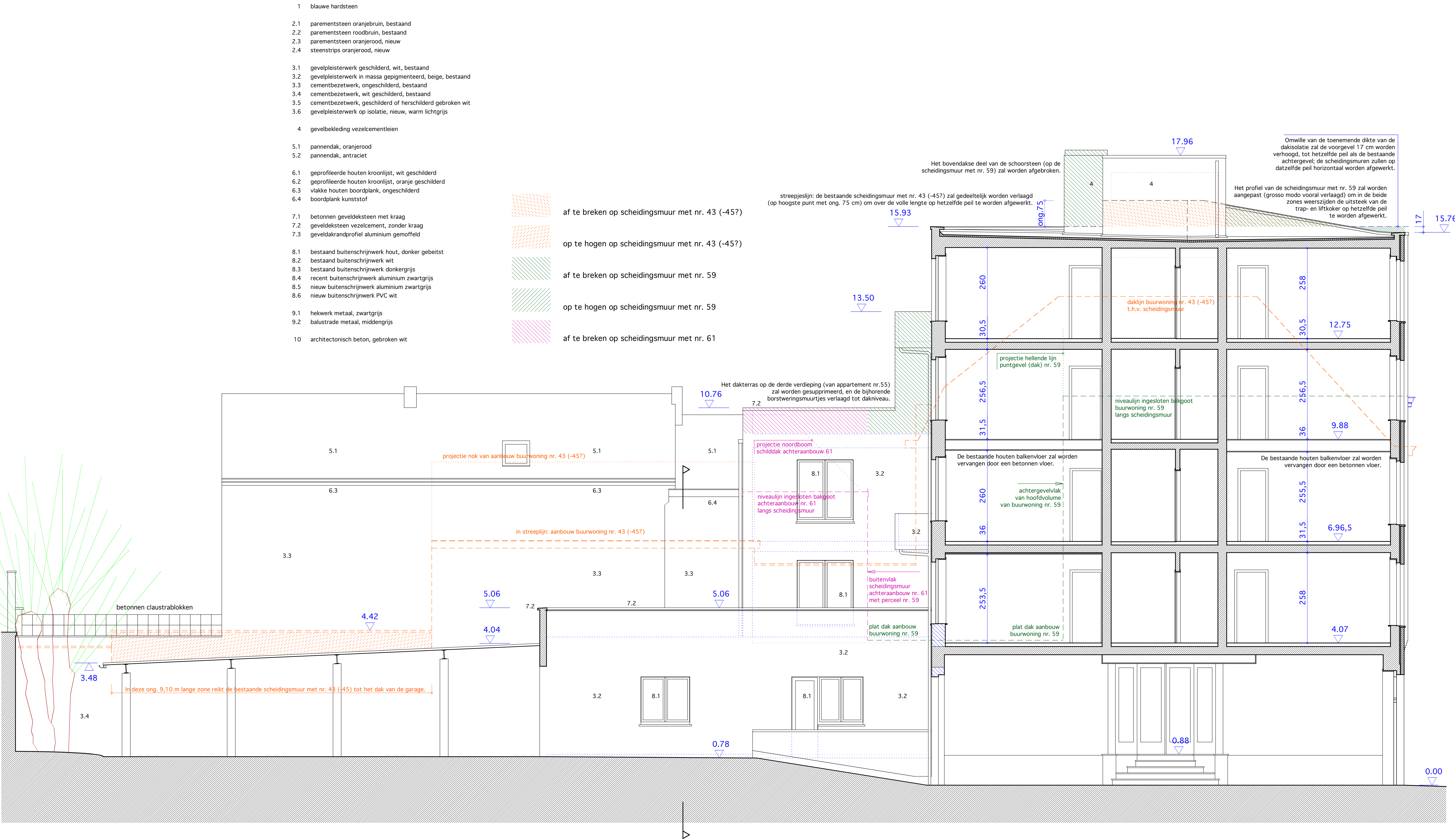
SLEEPSTRAAT (47-) 49-57, 9000 GENT * 1/50 DWARSDOORSNEDE t.h.v. DOORRIT, BESTAANDE TOESTAND
