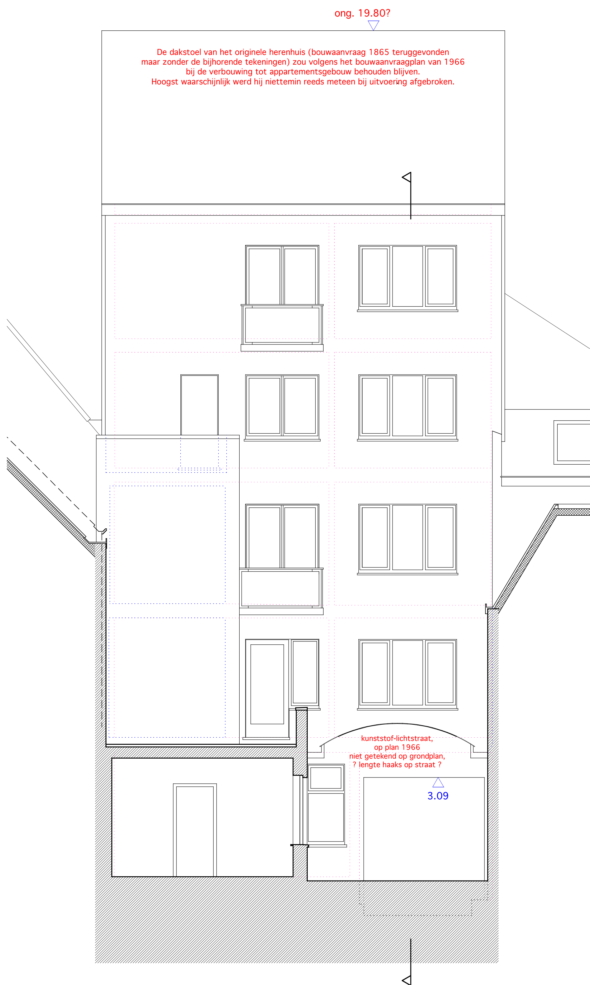
SLEEPSTRAAT (47-) 49-57, 9000 GENT 1/50 ACHTERGEVEL, SIMULATIE van VERGUNDE TOESTAND
