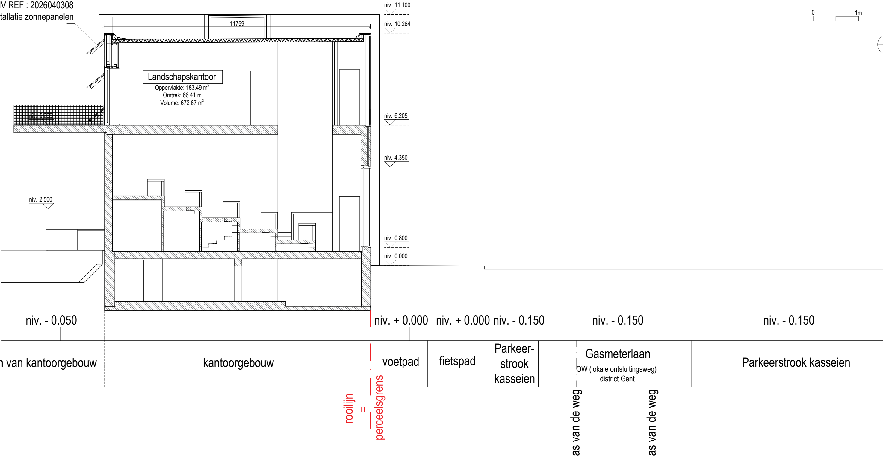
TERREINSNEDE A-A' BESTAANDE TOESTAND A3 schaal 1:100
