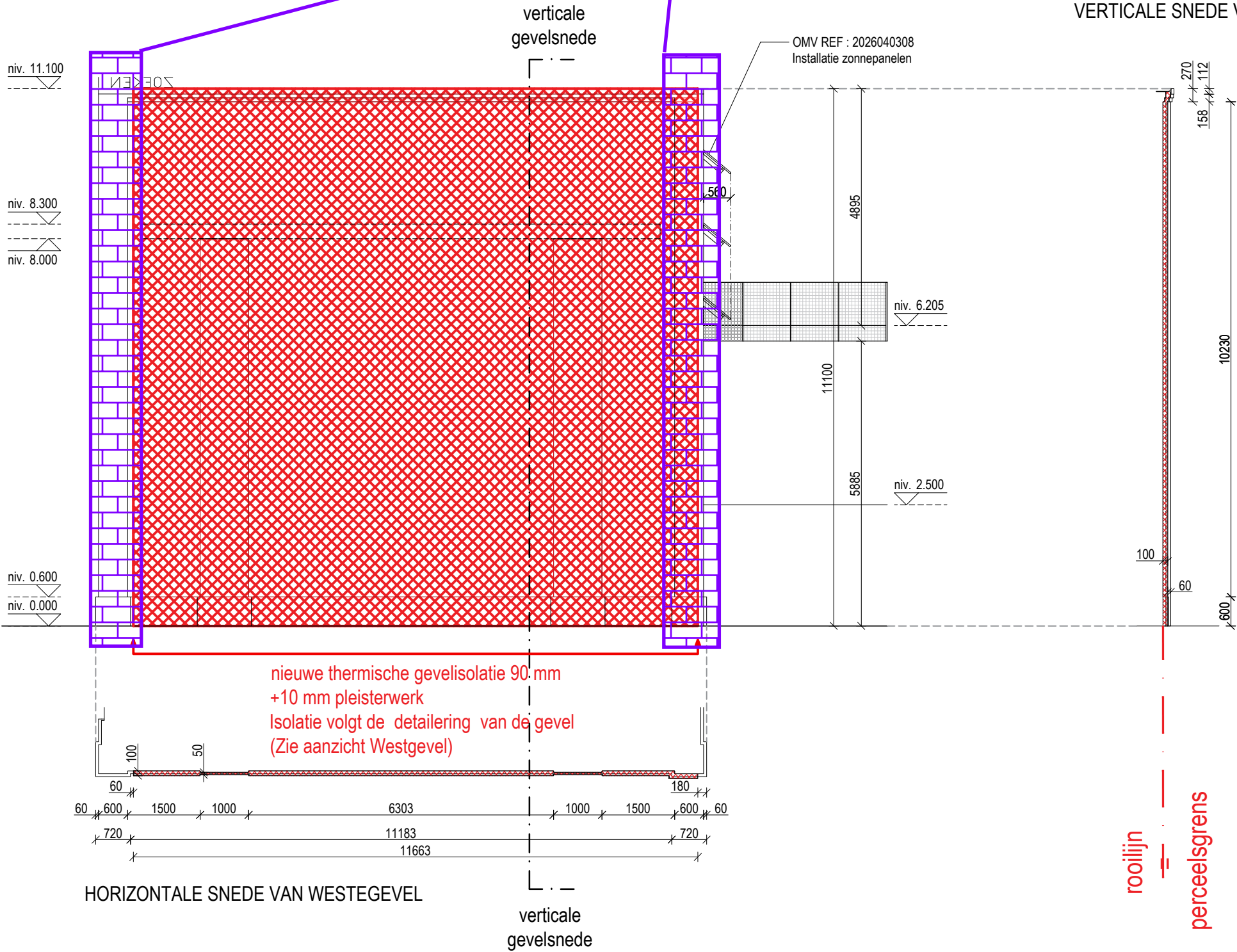
AANZICHT VAN WESTEGEVEL
