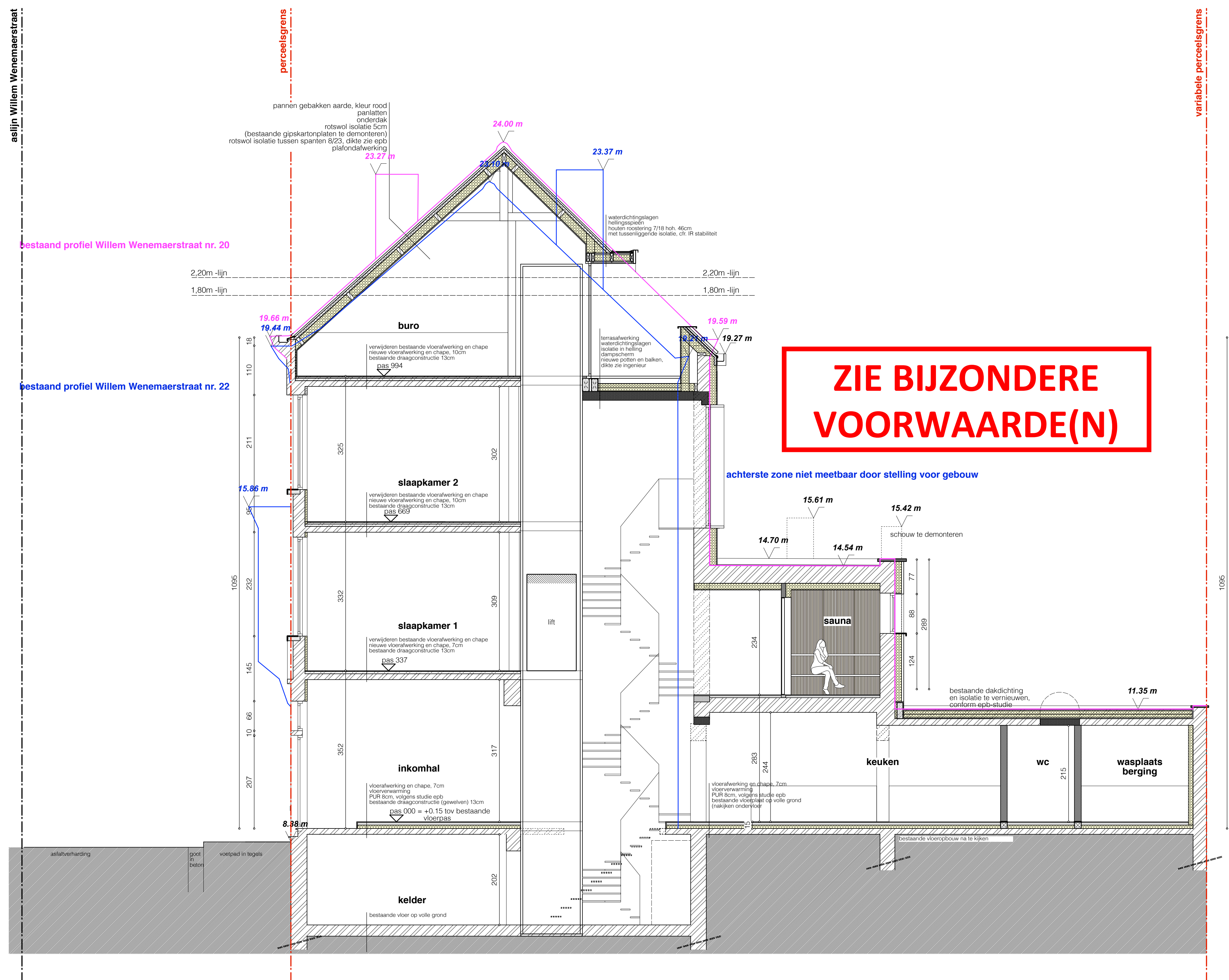
nieuwe toestand - Doorsnede BB schaal 1:50
