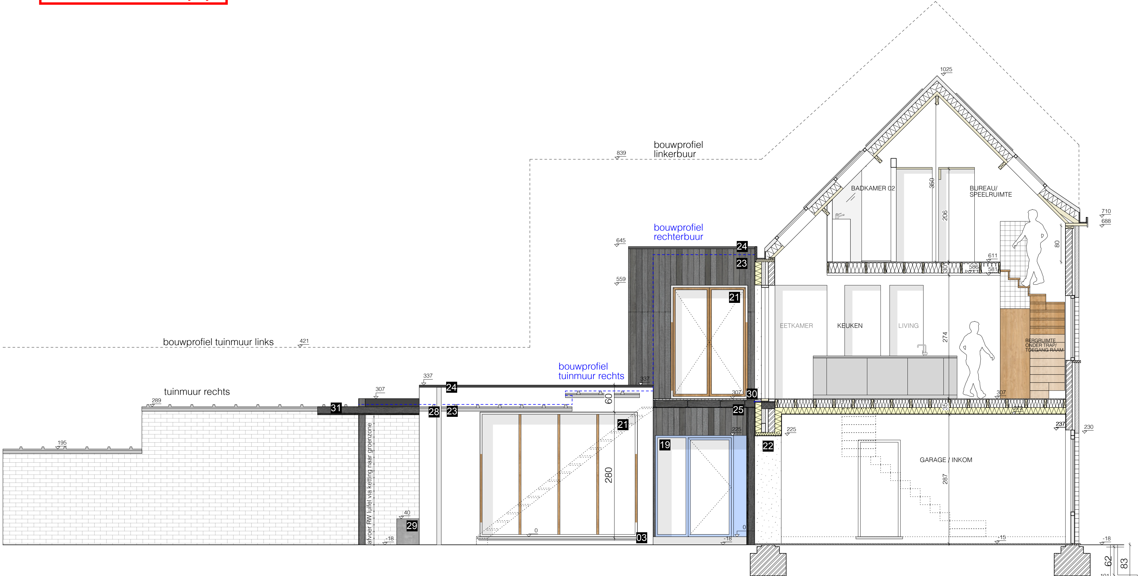
SNEDE AA' schaal 1/50 - meeteenheid cm
