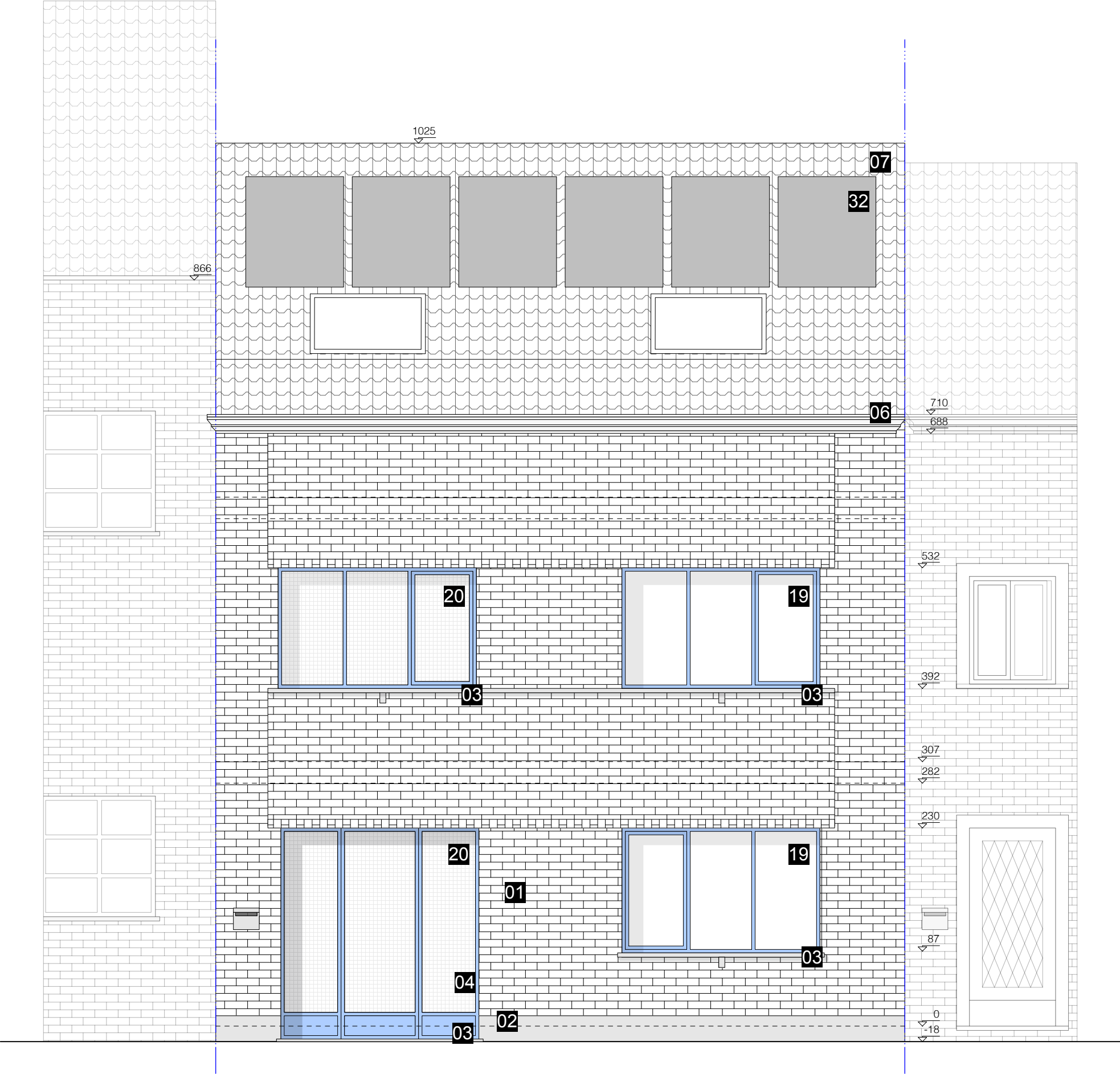
VOORGEVEL noordoost schaal 1/50 - meeteenheid cm
