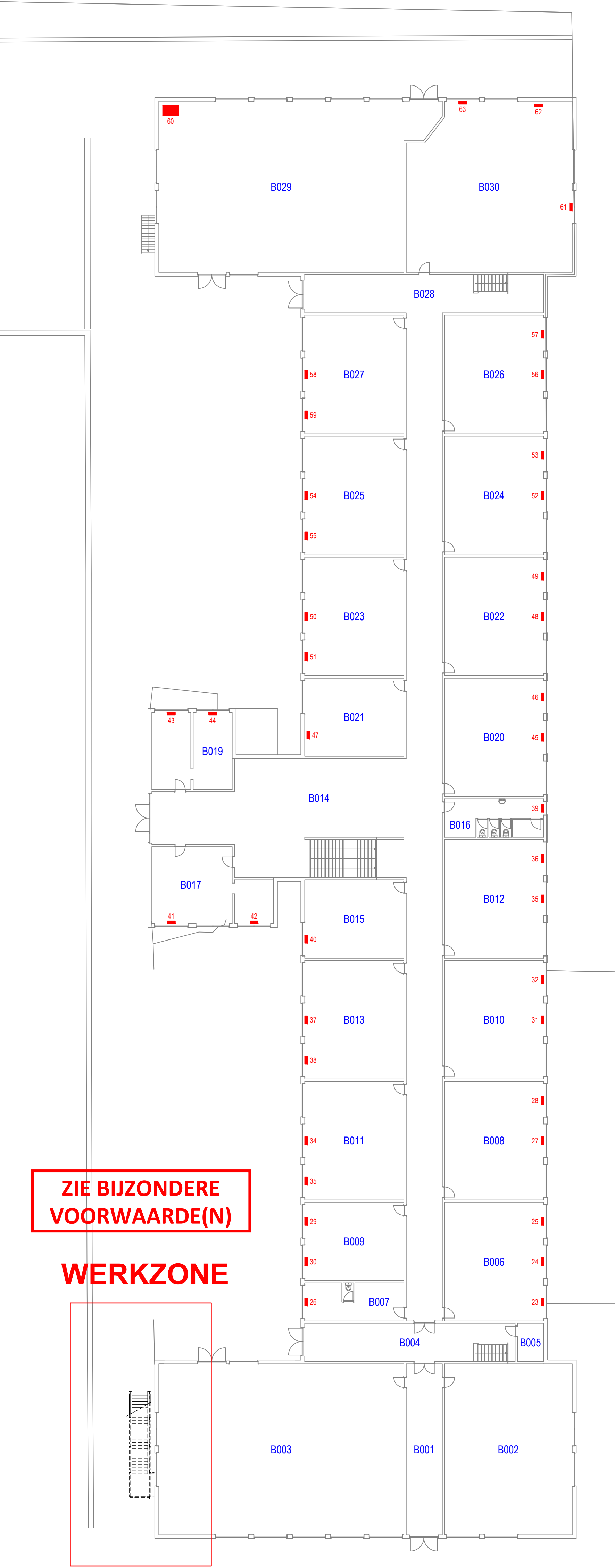
PLAN GELIJKVLOERS, nieuwe toestand schaal 1/200, maataanduidingen in meter.
