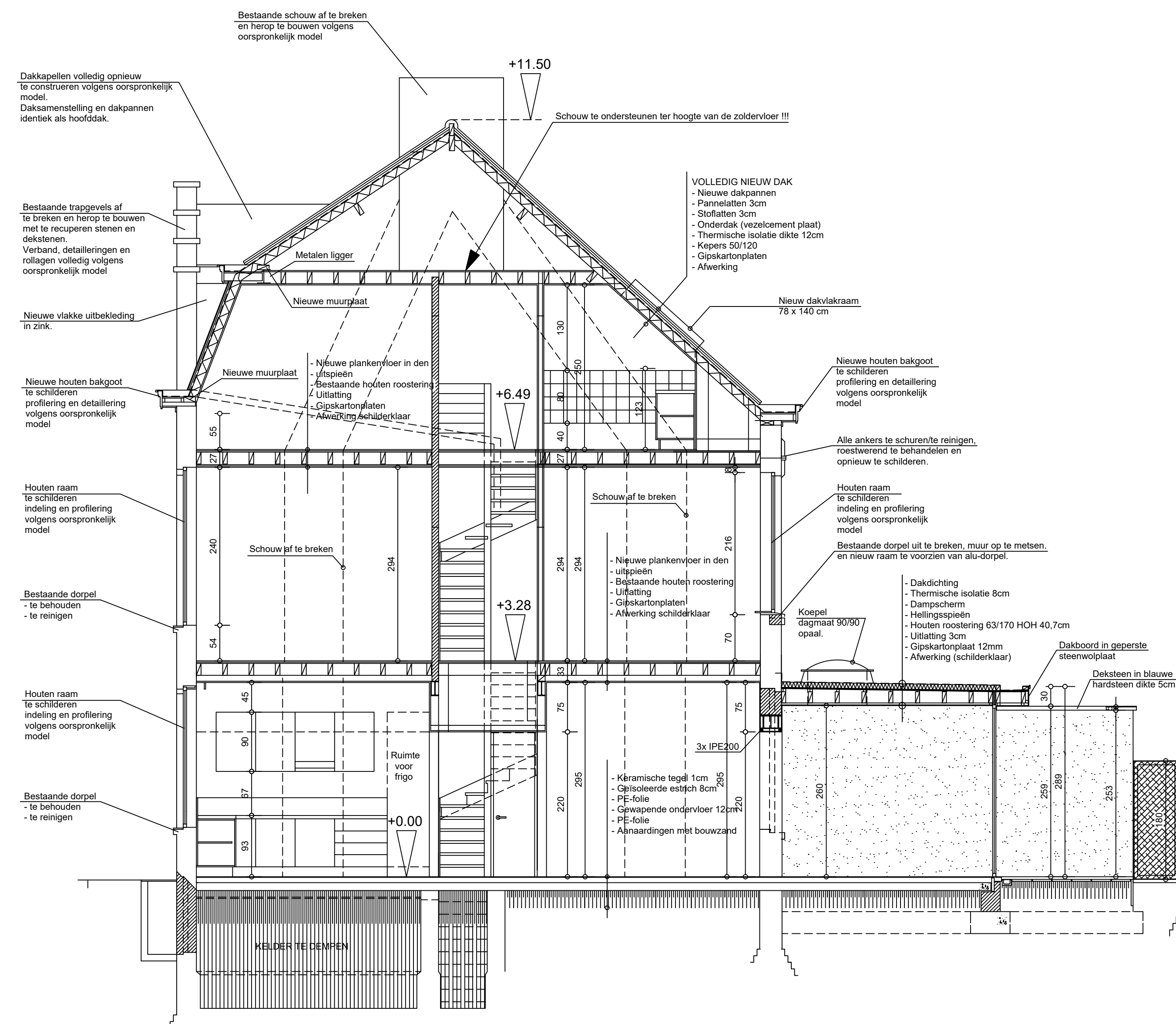
DOORSNEDE AA'
