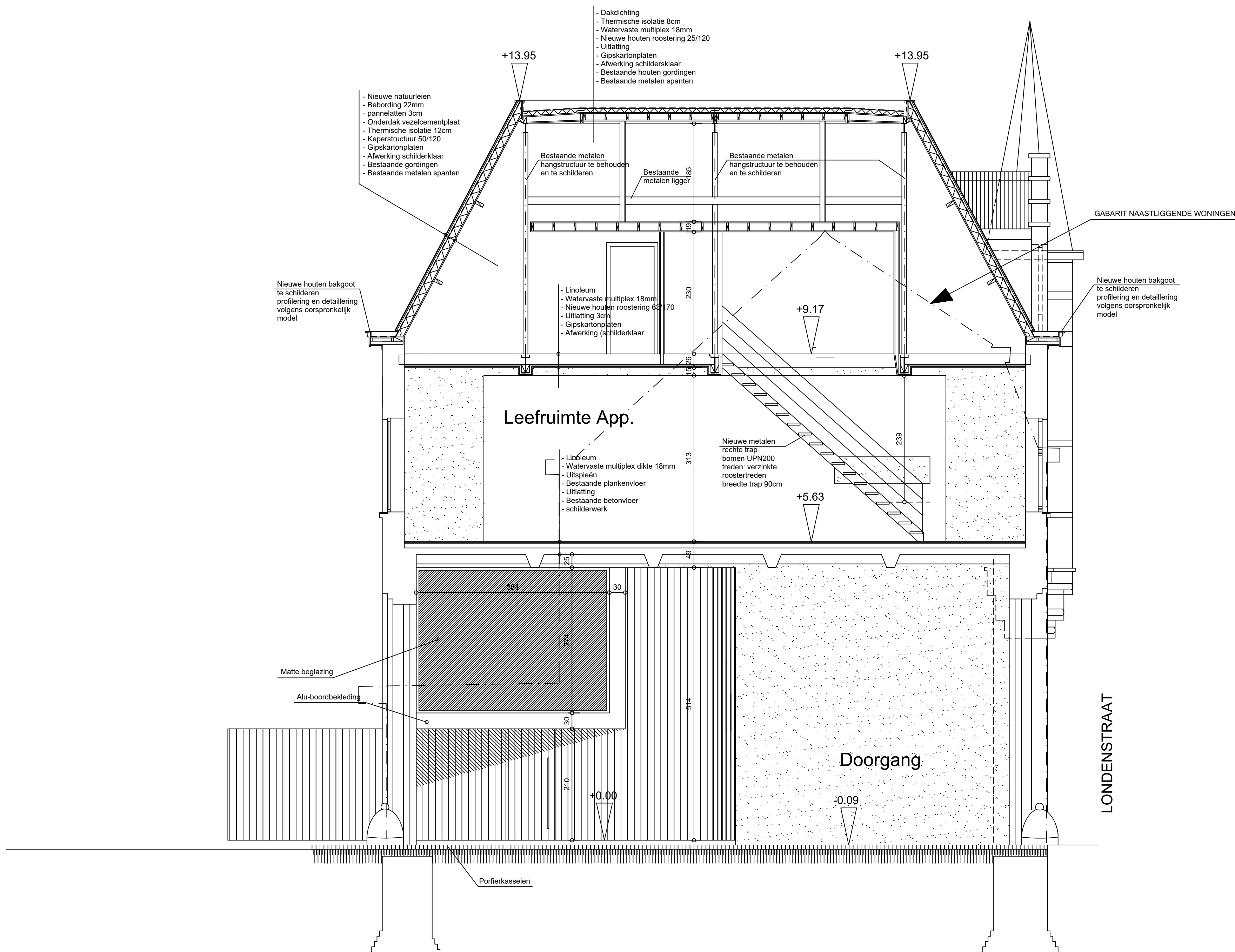
DOORSNEDE DD'
