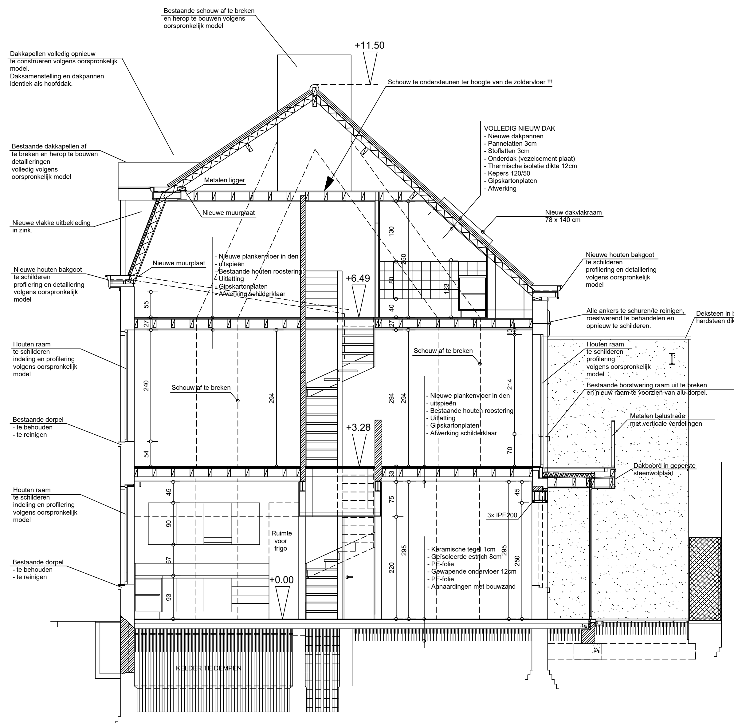
DOORSNEDE BB'
