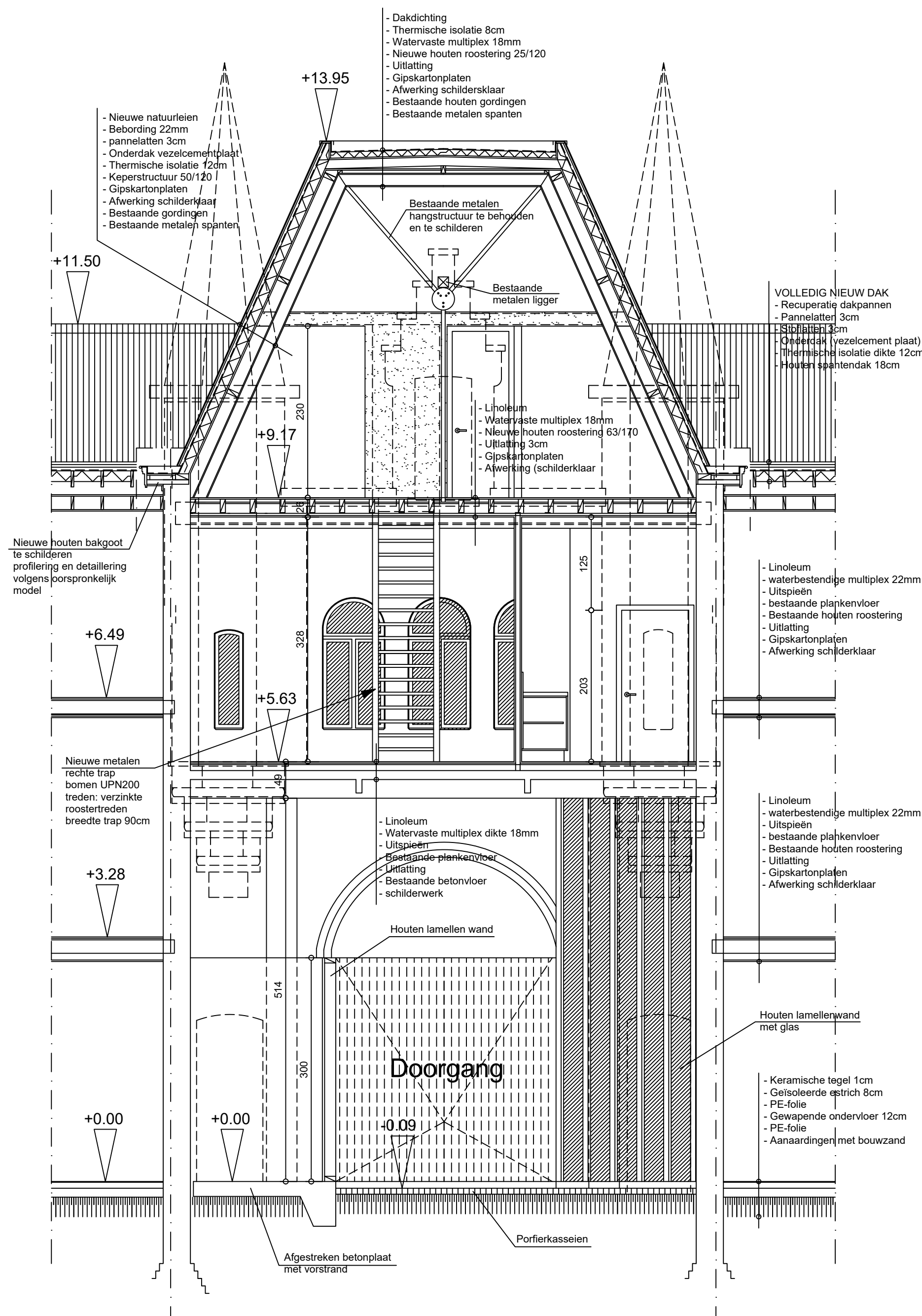
DOORSNEDE CC'
