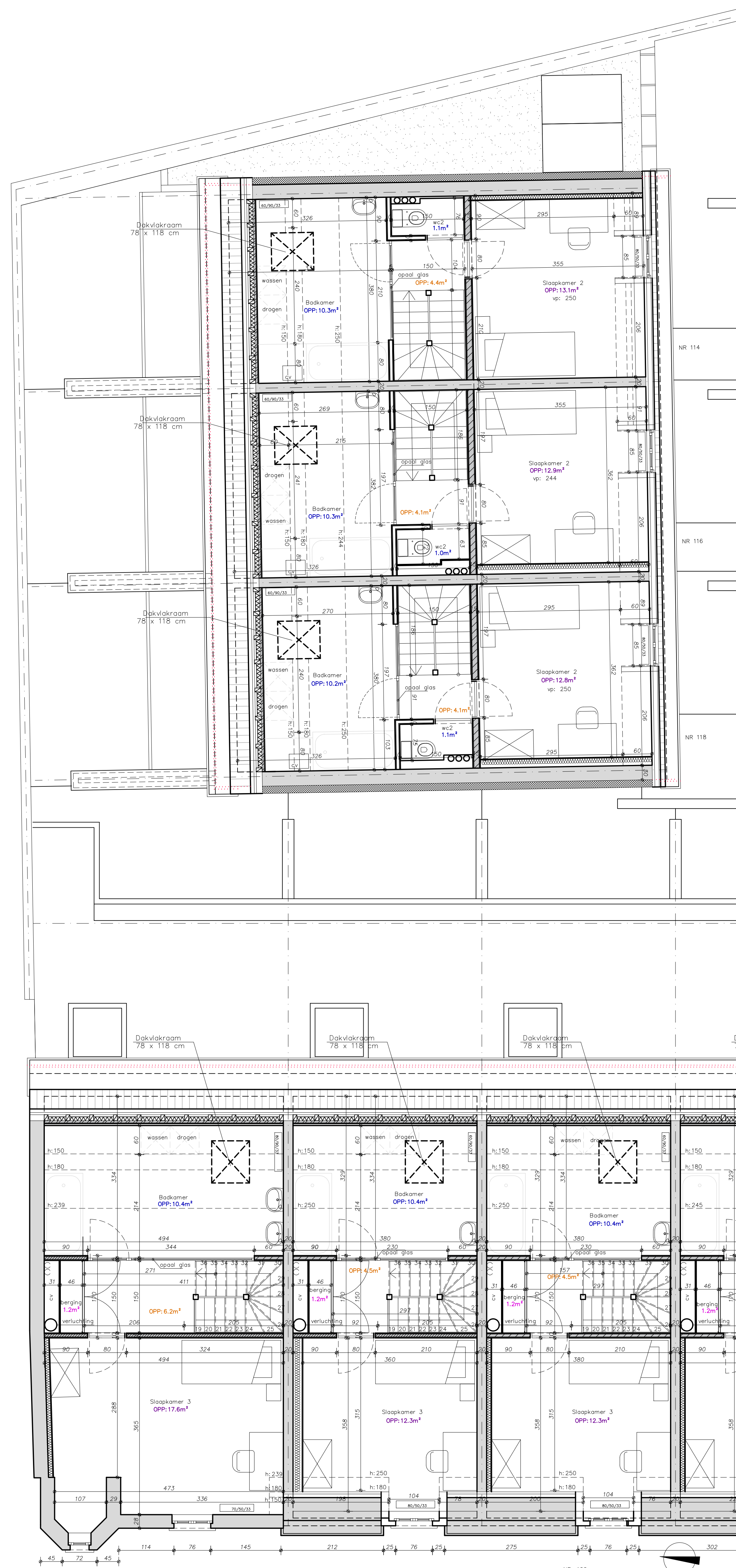
GRONDPLAN D verdieping +2 NIEUWE TOESTAND
