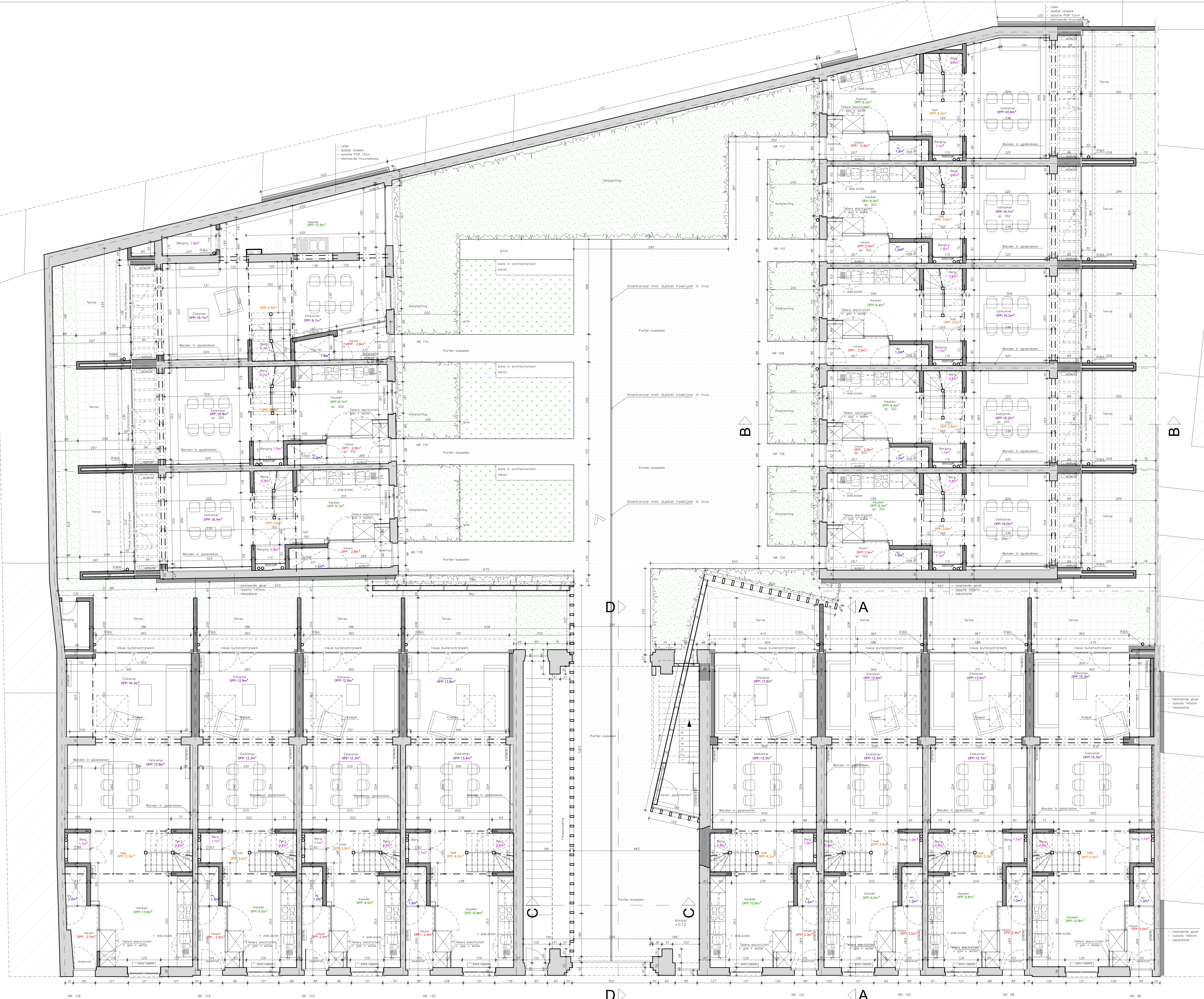
GRONDPLAN D gelijkvloers NIEUWE TOESTAND
