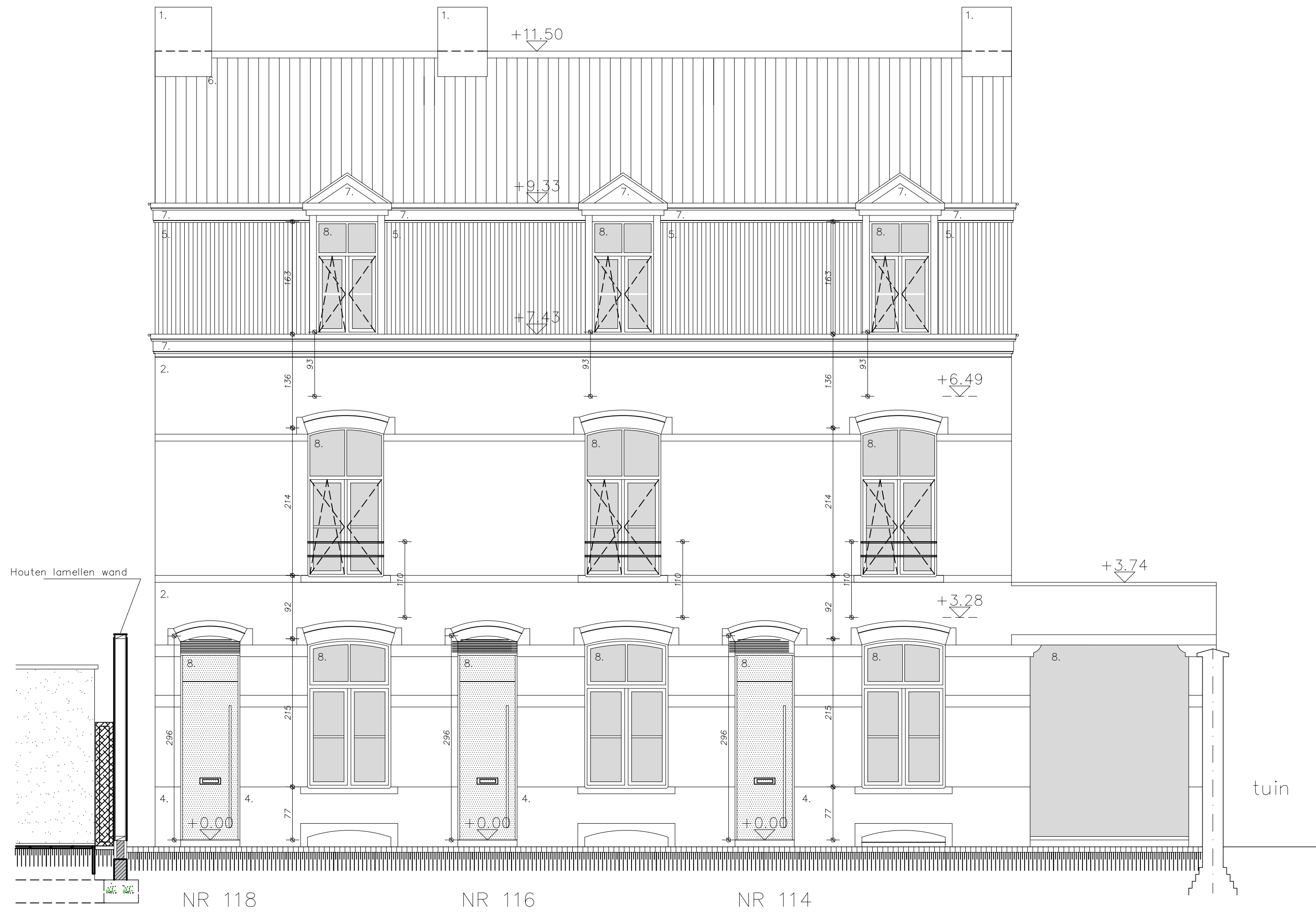
VOORGEVEL C binnenplein BESTAANDE TOESTAND
