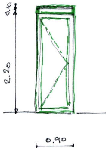
AANZICHT SNEDE CC
