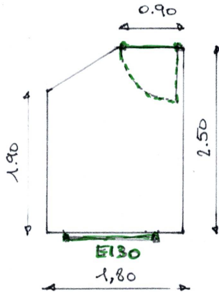
GRONDPLAN
