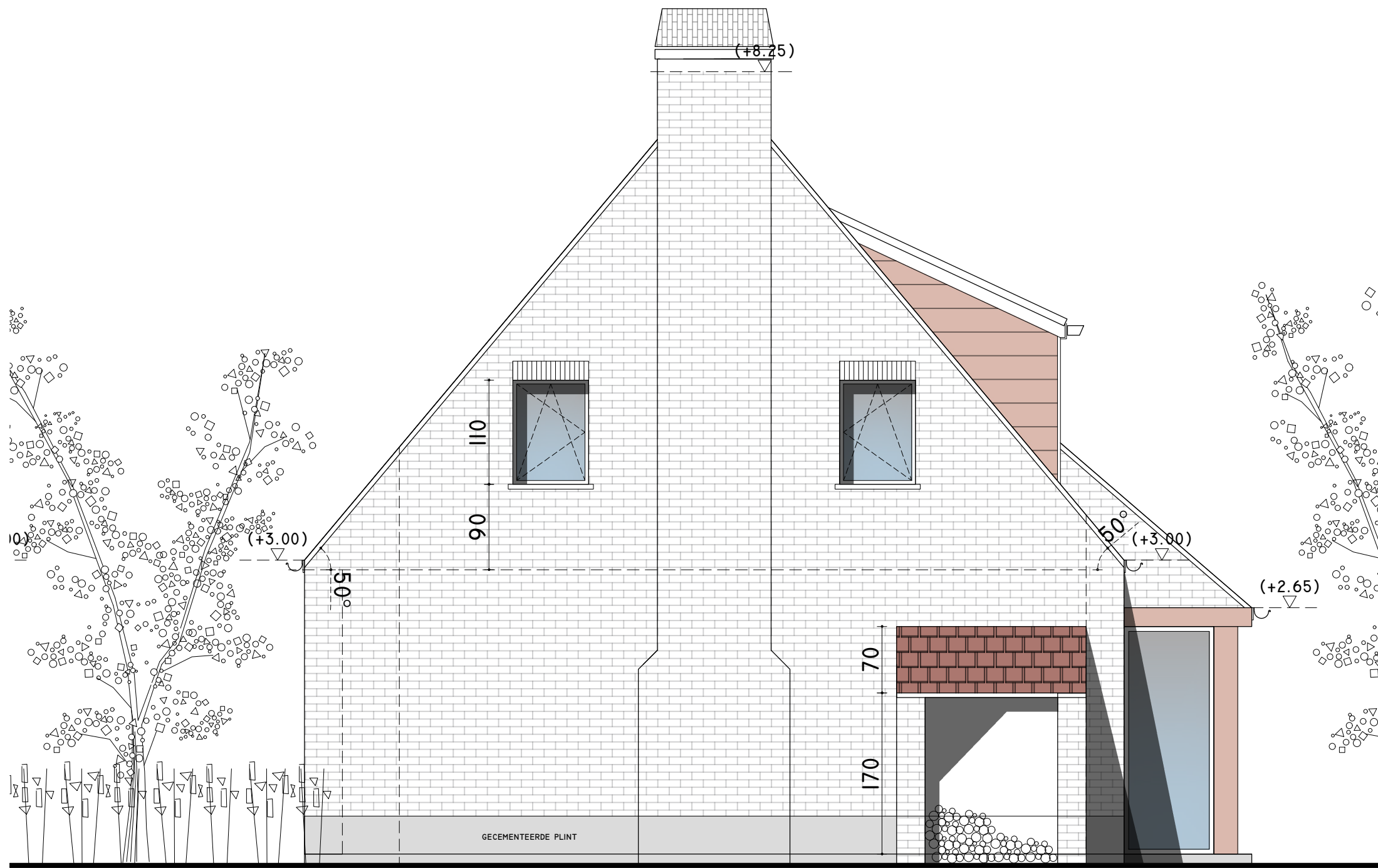
ZIJGEVEL RECHTS
