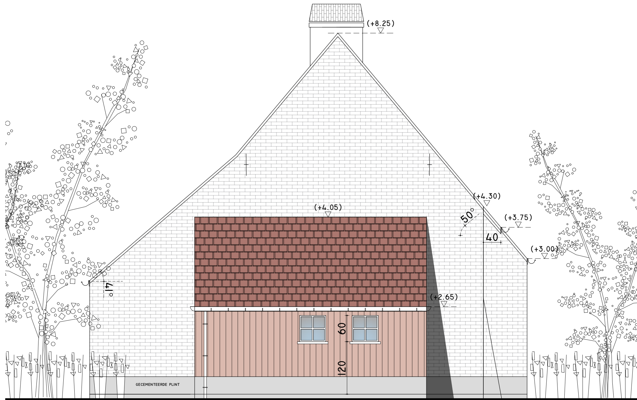
ZIJGEVEL LINKS
