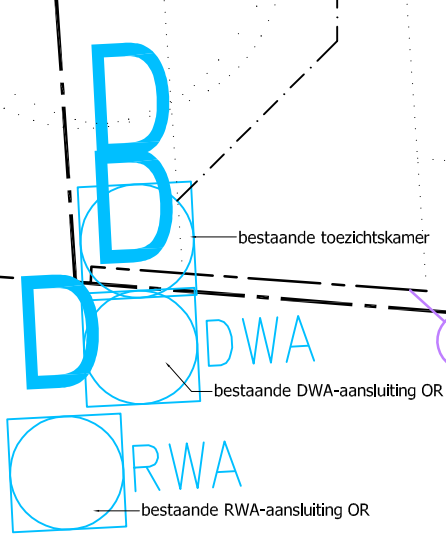
FUNDERINGS- & RIOLERINGSPLAN vergunde toestand - schaal 1:50
