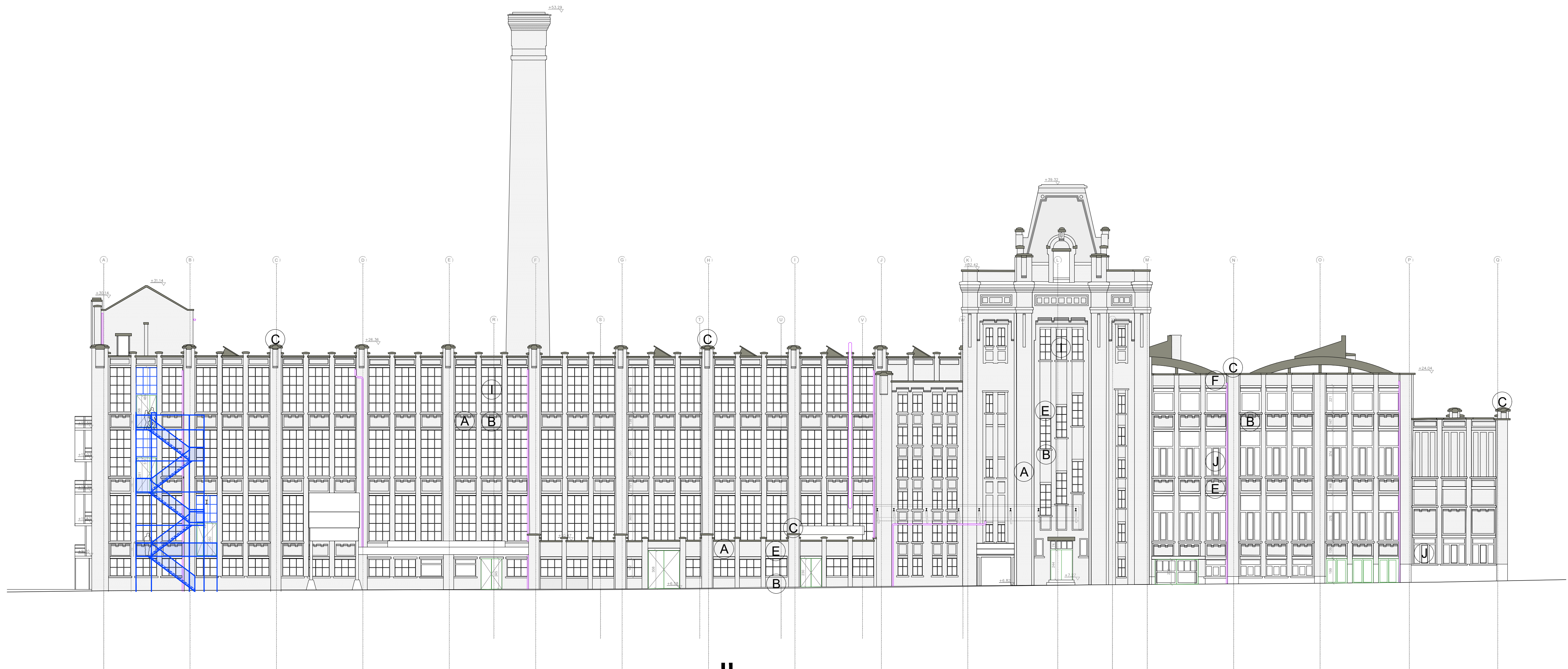
LINKERGEVEL (WEST) - NIEUWE TOESTAND - 1/200 -
